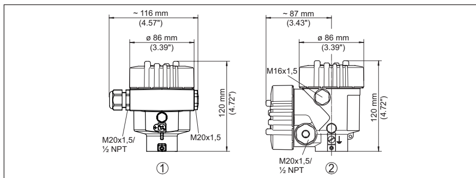
Fig. 45: Variantes da caixa com grau de proteção IP66/IP68 (0,2 bar), (com o módulo de visualização e configuração montado, a altura da caixa é aumentada em 9 mm/0,35 in)
