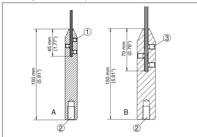
Fig. 34: Encurtar a sonda de medição com cabo
