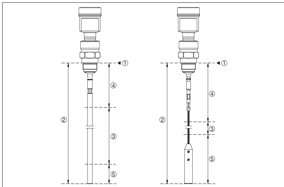
Fig. 39: Faixas de medição - VEGAFLEX 82
