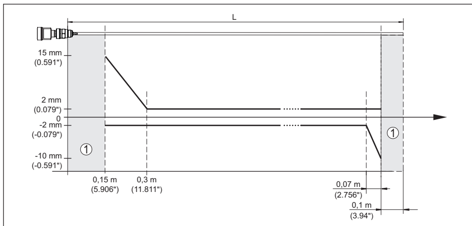
Fig. 40: Diferença de medição VEGAFLEX 82 em modelo com haste
