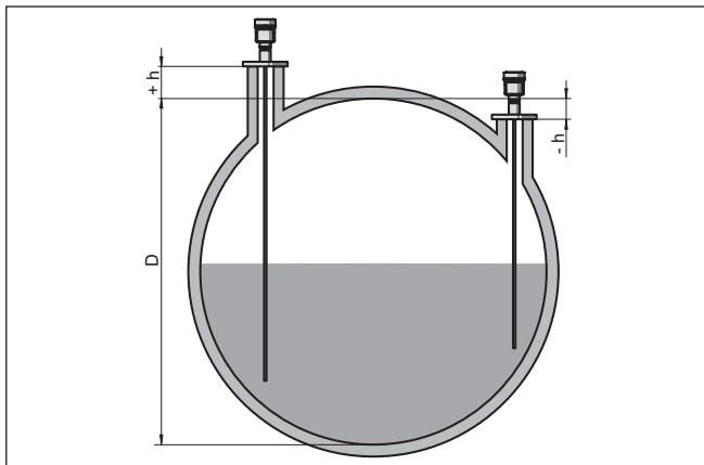
Fig. 24: Altura do reservatório e valor de correção da luva
