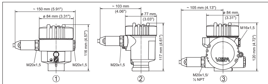
Fig. 48: Variantes da caixa com classe de proteção contra corpos estranhos e umidade IP66/IP68 (1 bar), (com módulo de visualização e configuração montado, a altura da caixa é aumentada em 9 mm/0,35 in)
