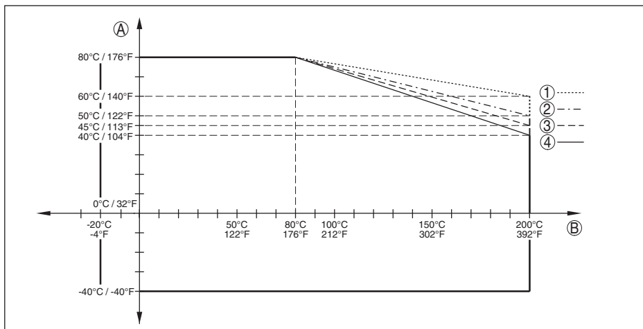
Fig. 43: Temperatura ambiente - Temperatura do processo, modelo com adaptador de temperatura
