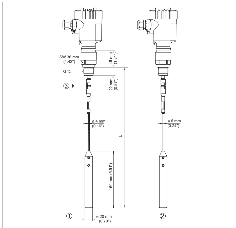
Fig. 49: VEGAFLEX 82, cabo de aço \varnothing 4 mm (0.157 in), \varnothing 6 mm (0.236 in) modelo com rosca com peso tensor (todos os pesos tensores com rosca M12 para olhal)
