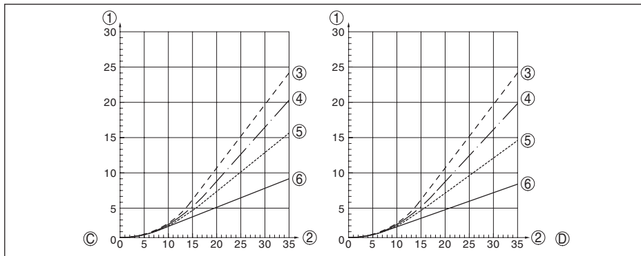
Fig. 38: Tração máxima no caso de areia e cimento - Cabo de aço: \phi 6 mm, \phi 11 mm, Revestido de PA
