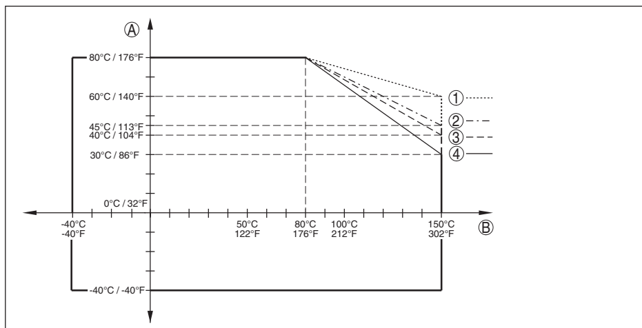
Fig. 42: Temperatura ambiente - Temperatura do processo, modelo padrão
