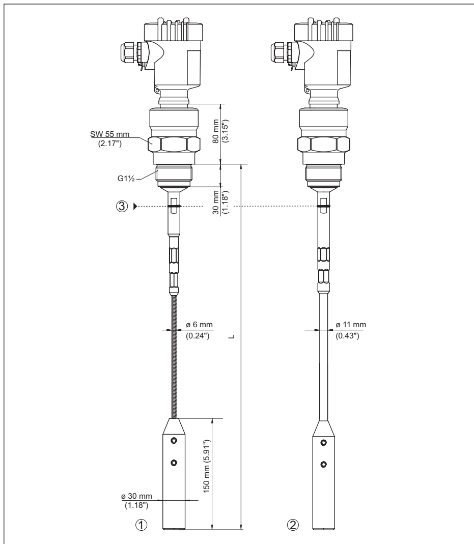
Fig. 50: VEGAFLEX 82, cabo de aço \varnothing 6 mm (0.236 in), \varnothing 11 mm (0.433 in) modelo com rosca com peso tensor (todos os pesos tensores com rosca M12 para olhal)
