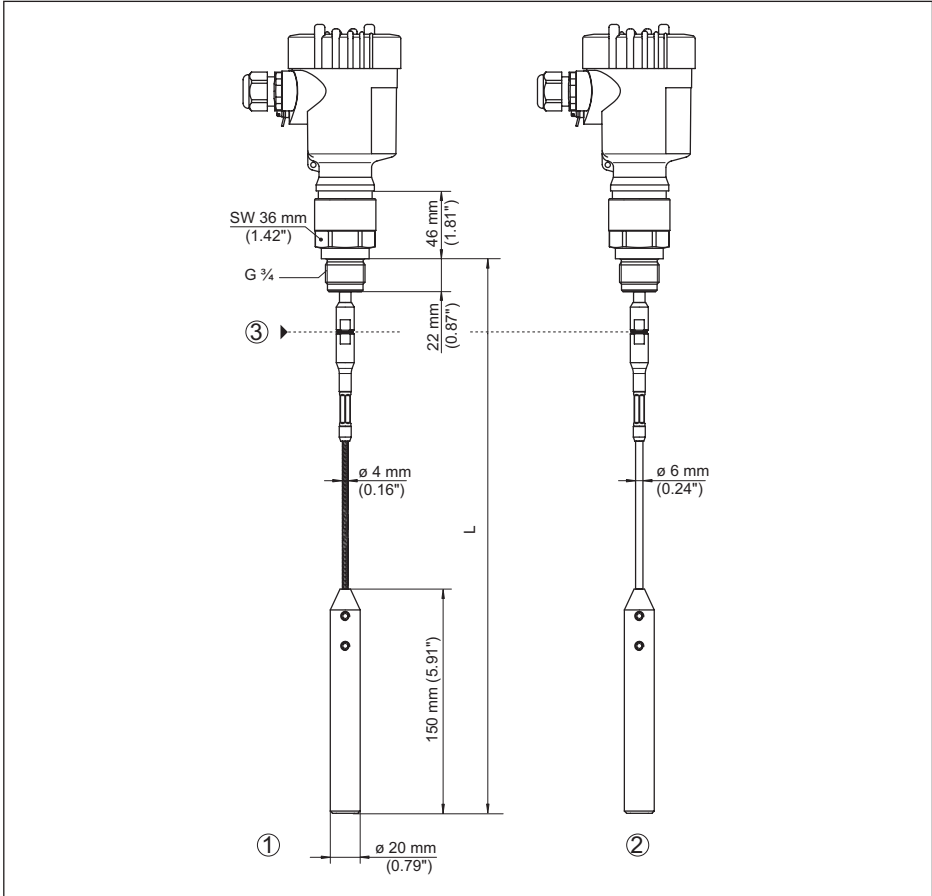
Fig. 49: VEGAFLEX 82, kabel \varnothing 4 mm (0.157 in), \varnothing 6 mm (0.236 in) schroefdraaduitvoering met spangewicht (alle spangewichten met schroefdraad M12 voor oogbout)
