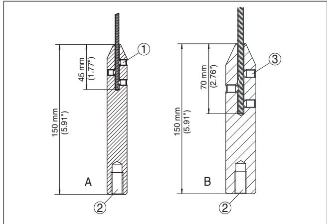
Fig. 34: Kabelmeetsonde inkorten
