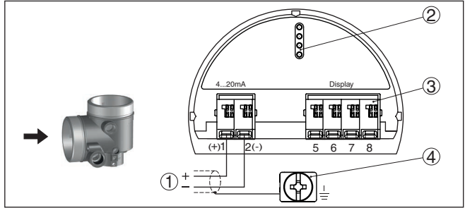
Fig. 12: Aansluitruimte - tweekamerbehuizing
