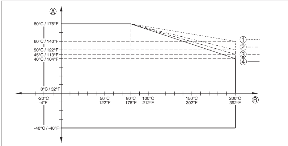
Fig. 43: Omgevingstemperatuur - procestemperatuur, uitvoering met temperatuurtussenstuk
