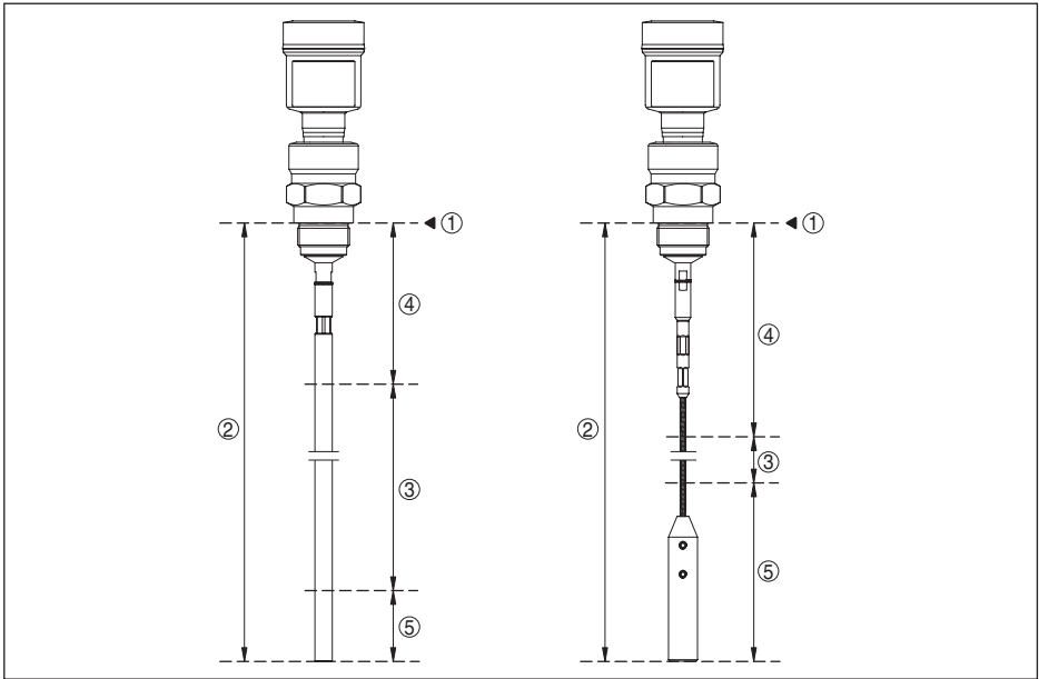
Fig. 39: Meetbereiken - VEGAFLEX 82
