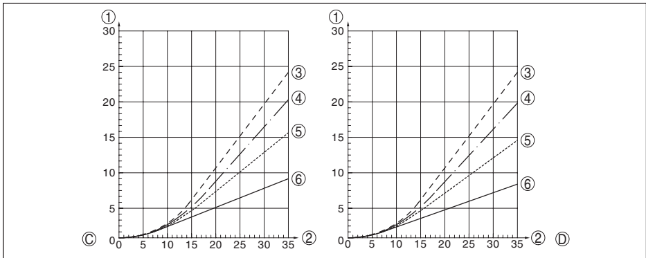
Fig. 38: Maximale trekbelasting bij zand en cement - kabel: \varnothing 6 mm, \varnothing 11 mm, PA-mantel
