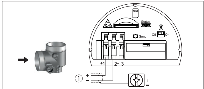
Fig. 13: Aansluitruimte - radiografische PLICSMOBILE 81
