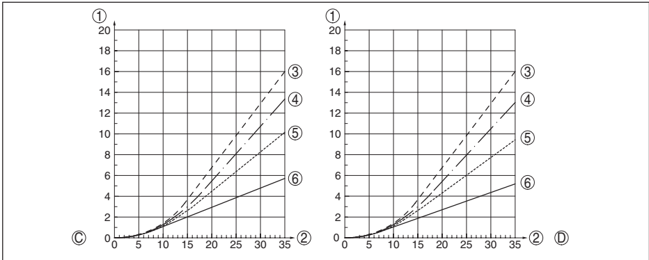
Fig. 36: Maximale trekbelasting bij zand en cement - kabel: \phi 4 mm (0.157 in)
