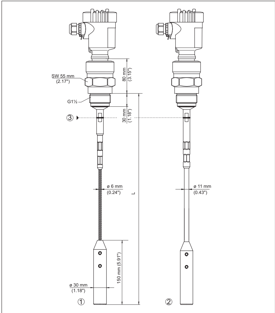
Fig. 50: VEGAFLEX 82, kabel \varnothing 6 mm (0.236 in), \varnothing 11 mm (0.433 in) schroefdraaduitvoering met spangewicht (alle spangewichten met schroefdraad M12 voor oogbout)
