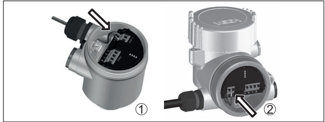
Fig. 9: Aansluitstappen 5 en 6
