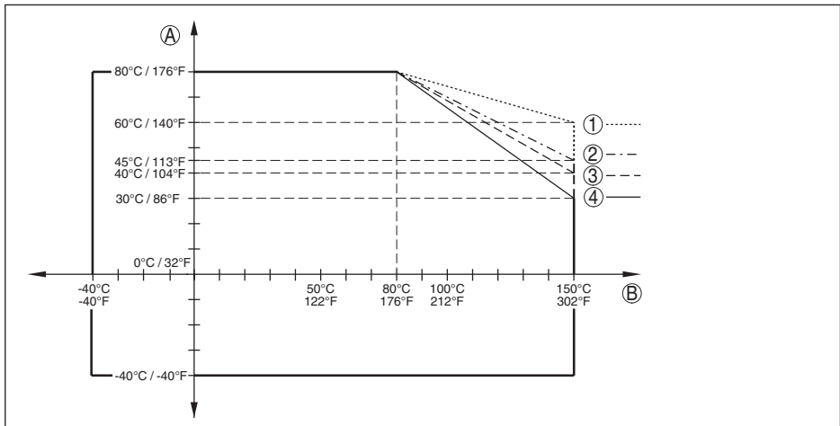
Fig. 42: Omgevingstemperatuur - procestemperatuur standaarduitvoering
