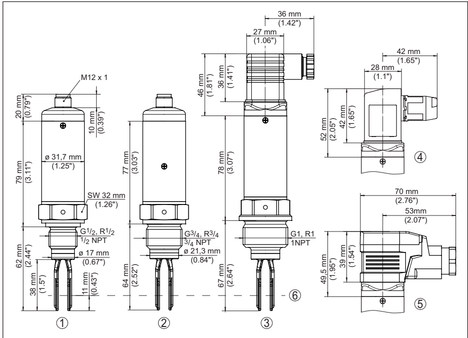
Fig. 18: VEGASWING 51, Versión alta temperatura - Conexiones roscadas
