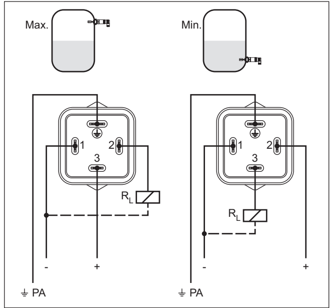
Fig. 12: Esquema de conexión, salida de transistor para enchufe de válvula DIN 4400
