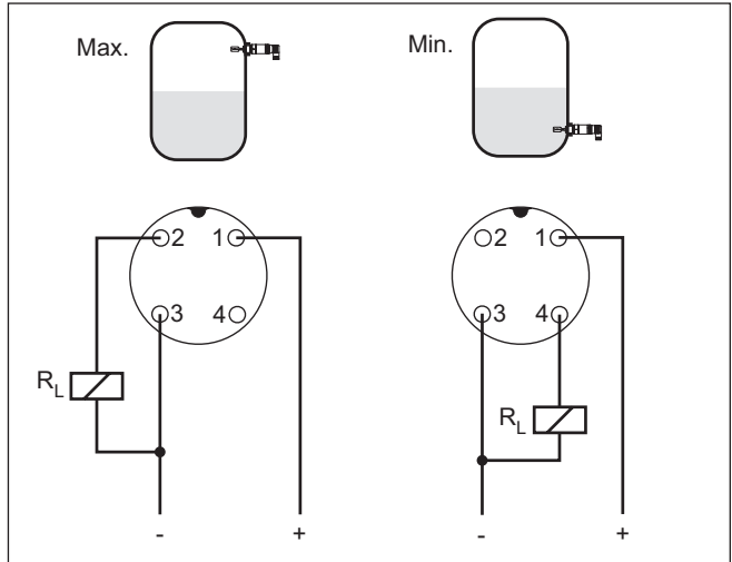
Fig. 13: Esquema de conexión (carcasa), salida de transistores de la conexión de enchufe M12 x 1
