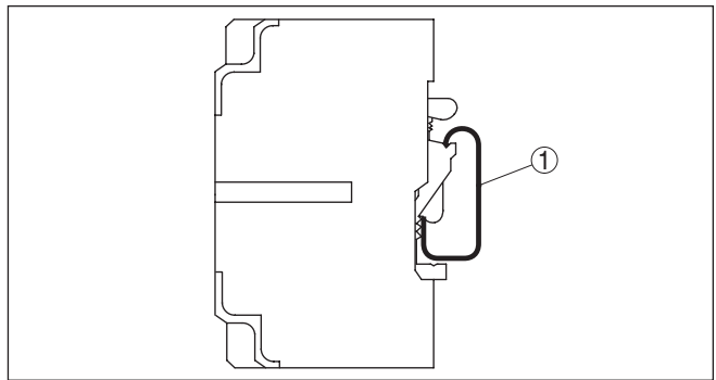
Fig. 3: Montagem em trilho de fixação conforme EN 50 035 (trilho com perfil C) 35 x 7,5 mm
