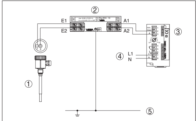
Fig. 8: Esquema de ligações B53-19 com sonda de medição capacitiva de uma haste
