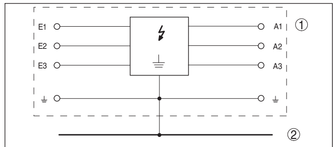
Fig. 7: Diagrama de circuitos B53-19
