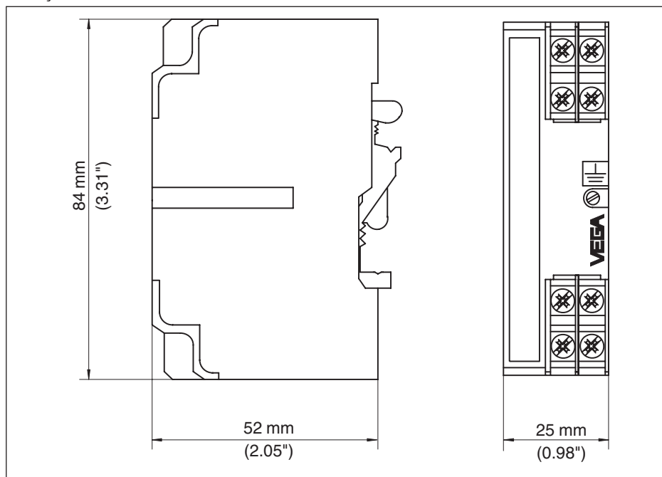
Fig. 10: Dimensões B53-19
