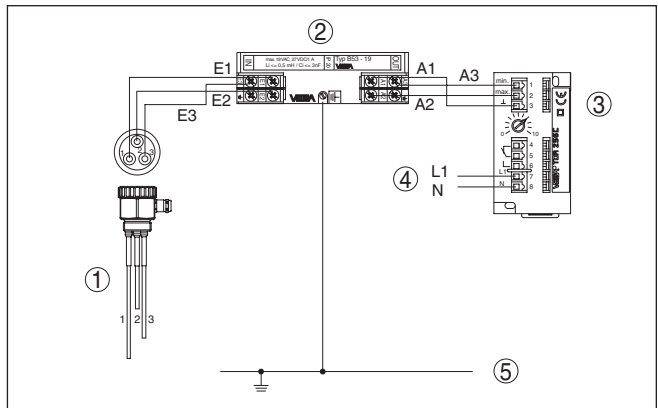
Fig. 9: Esquema de ligações B53-19 com sonda de medição capacitiva de três hastas
