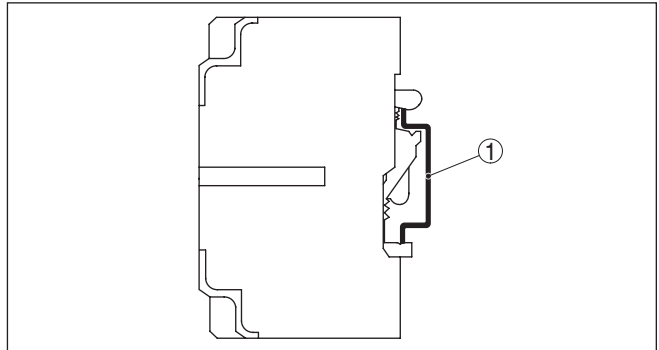
Fig. 2: Montagem em trilho de fixação conforme EN 50 022 (trilho DIN) 35 x 7,5 mm
