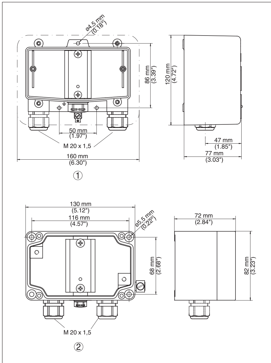
Fig. 11: Dimensões B53-19
