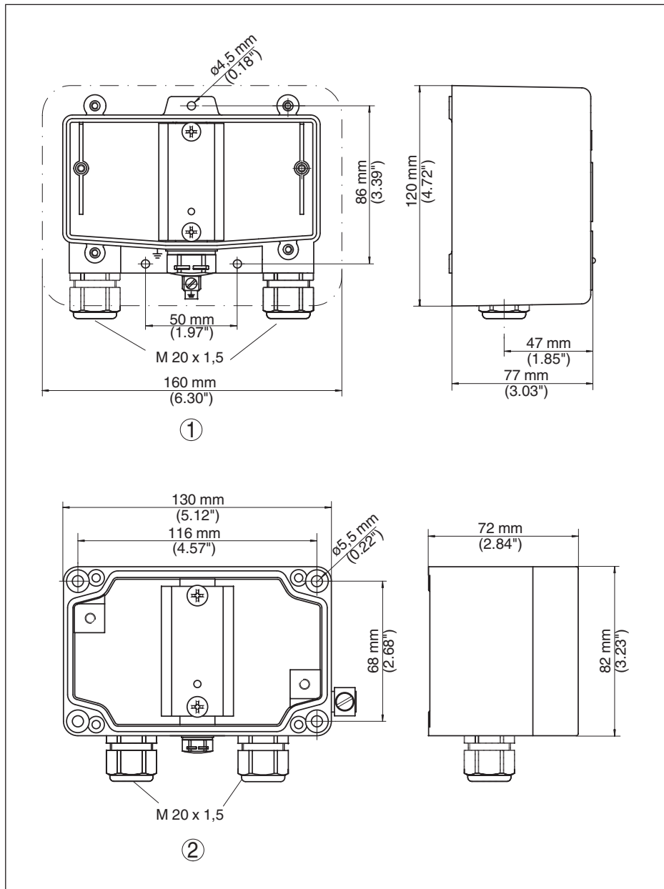
Fig. 11: Encombrement B53-19
