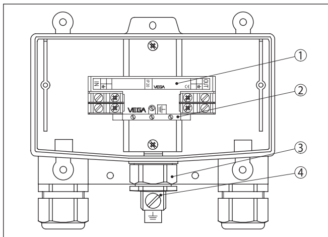
Fig. 6: Montaje en carcasa plástica
