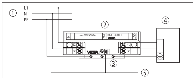
Fig. 8: Esquema de conexiones del aparato de protección contra sobretensión B61-300 FI dentro de la carcasa
