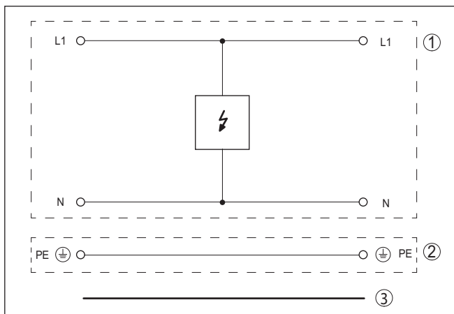
Fig. 7: Diagrama de circuitos aparato de protección contra sobretensiones B61-300 FI
