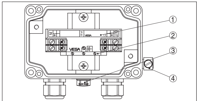
Fig. 5: Montaje en carcasa de aluminio
