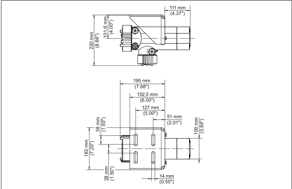
Abb. 28: POINTRAC 31 ohne Detektorrohr, 46 mm (1.8 in) - mit mitgeliefertem Montagezubehör
