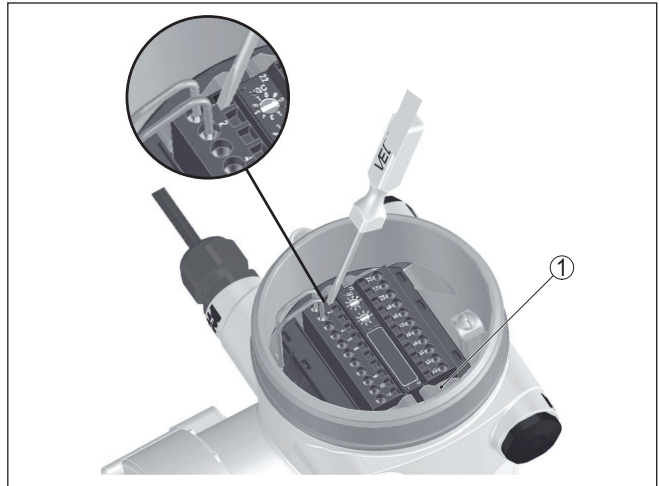
Abb. 11: Anschlusschritte 4 und 5
