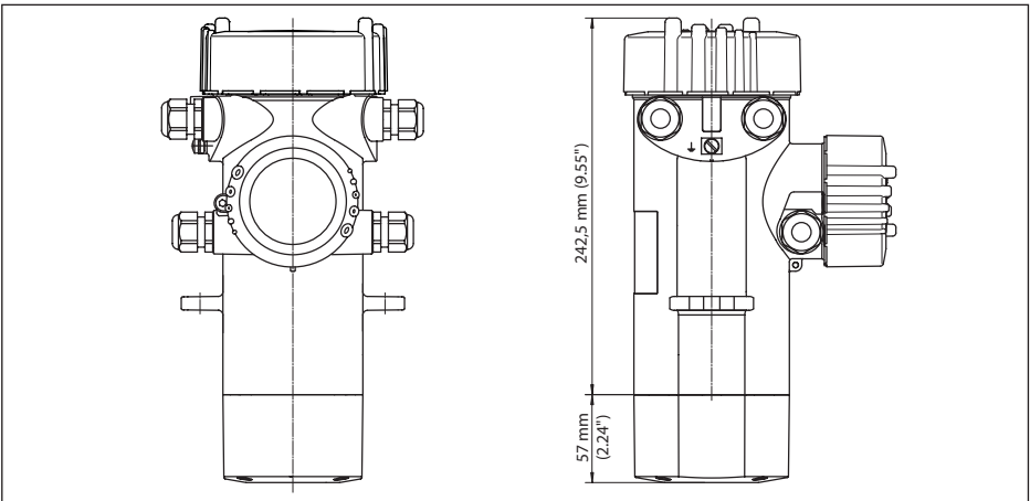
Abb. 27: POINTRAC 31 ohne Detektorrohr - Messbereich = Bestelllänge 46 mm (1.8 in)
