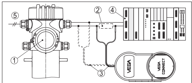
Abb. 20: Anschluss des PCs via HART an die Signalleitung
