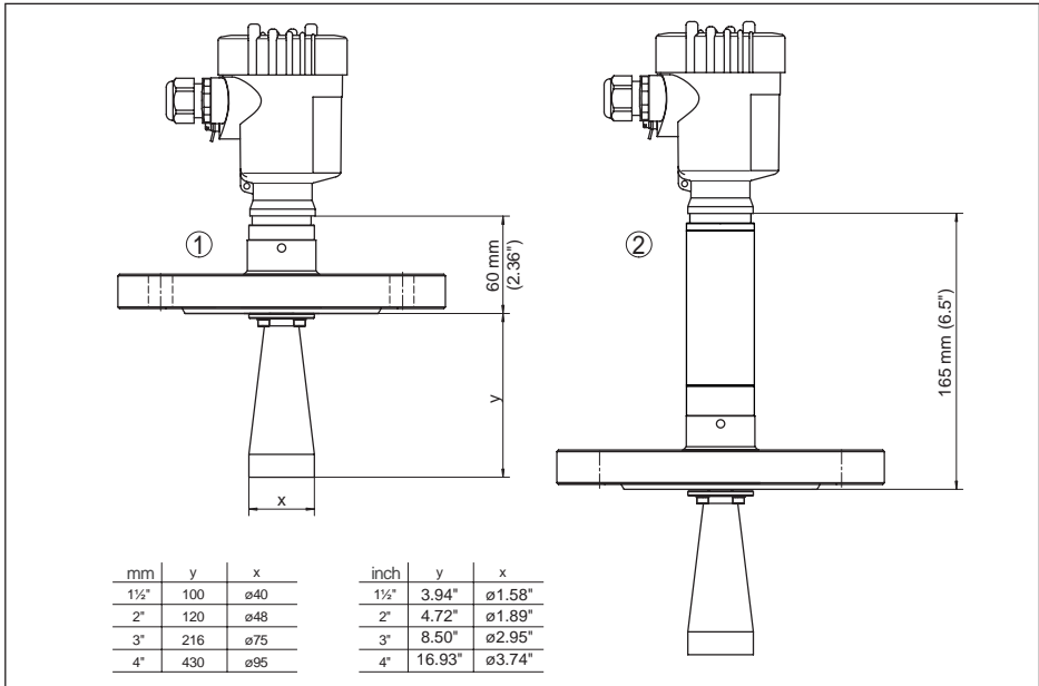
Figura 65: VEGAPULS 62, antenna a cono in esecuzione a flangia
