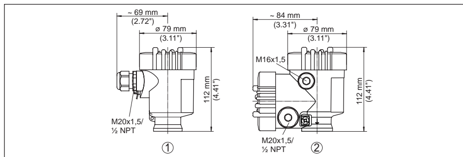
Figura 59: Le differenti custodie con grado di protezione IP 66/IP 67 (con tastierino di taratura con display incorporato l'altezza della custodia aumenta di 9 mm/0.35 in)
