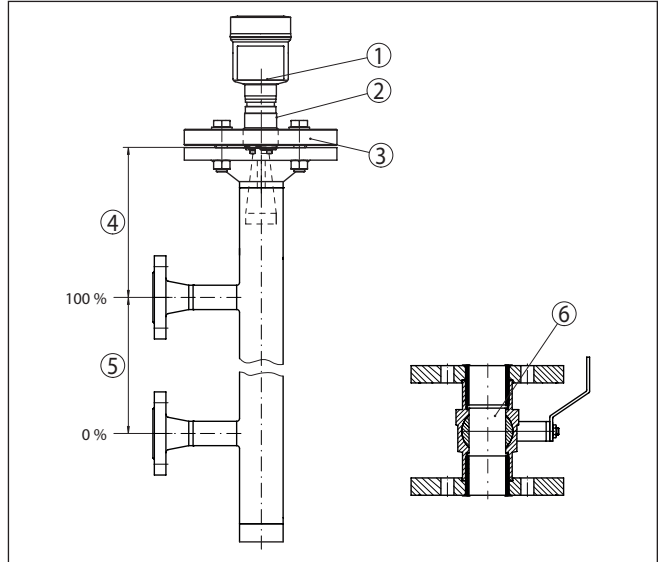
Figura 20: Struttura del bypass
