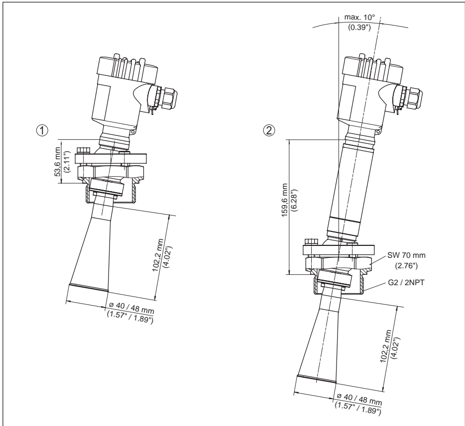
Figura 69: VEGAPULS 62, antenna a cono e supporto orientabile, attacco filettato
