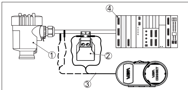
Figura 40: Collegamento del PC via HART alla linea del segnale
