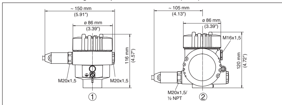
Figura 61: Differenti custodie con grado di protezione IP 66/IP 68 (1 bar), (con tastierino di taratura con display incorporato l'altezza della custodia aumenta di 18 mm/0.71 in)
