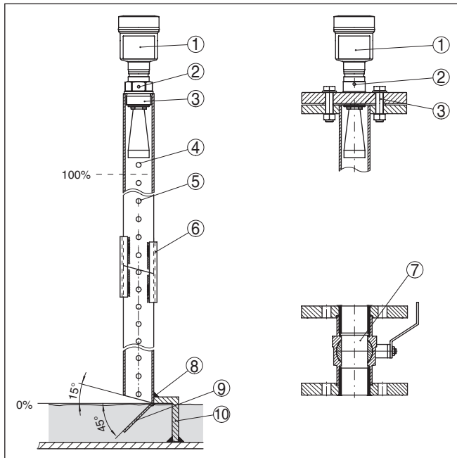
Figura 18: Struttura del tubo di calma VEGAPULS 62
