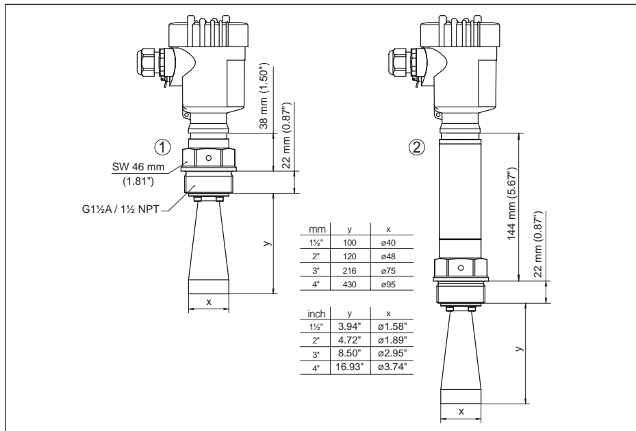
Figura 64: VEGAPULS 62, antenna a cono in esecuzione filettata
