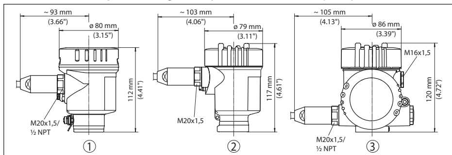
Figura 63: Differenti custodie con grado di protezione IP 66/IP 68 (1 bar), (con tastierino di taratura con display incorporato l'altezza della custodia aumenta di 18 mm/0.71 in)
