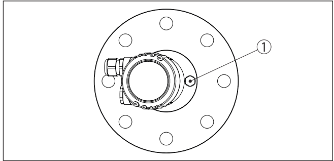
Figura 14: VEGAPULS 62 con supporto orientabile
