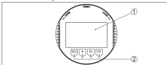
Figura 36: Elementi d'indicazione e di servizio
