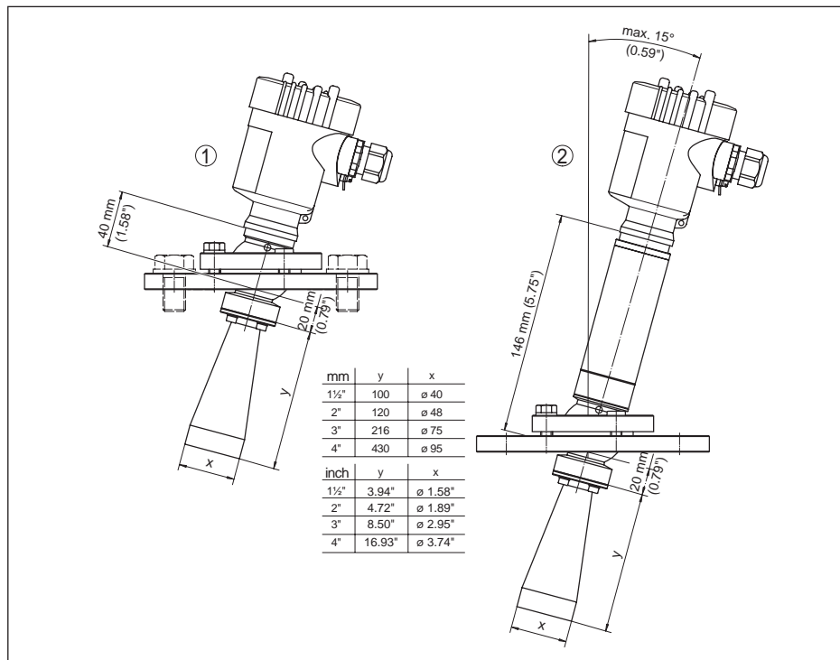
Figura 68: VEGAPULS 62, antenna a cono e supporto orientabile
