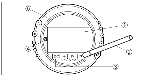
Figura 37: Elementi di visualizzazione e calibrazione - con calibrazione tramite penna magnetica
