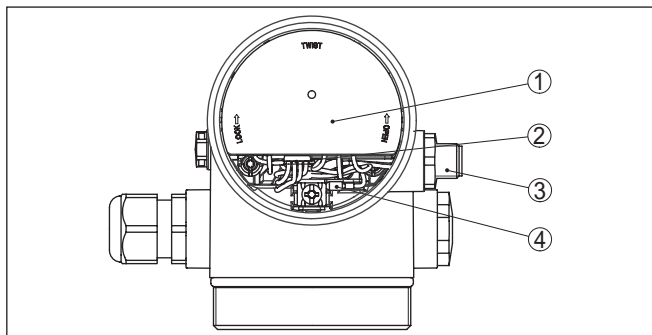
Figura 31: Vista sul vano dell'elettronica con adattatore VEGADIS per il collegamento dell'unità d'indicazione e di calibrazione esterna
