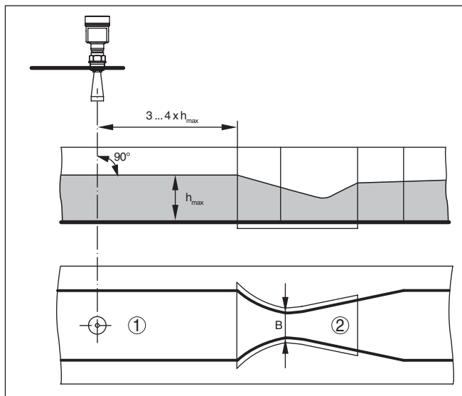
Figura 22: Misura di portata con canale Khafagi-Venturi: h_{max} = max. riempimento del canale; B = massima strozzatura del canale
