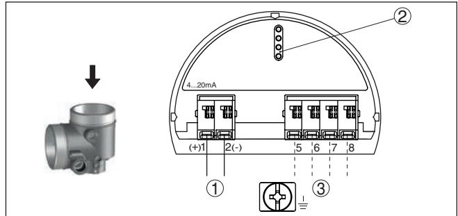
Figura 28: Vano dell'elettronica - custodia a due camere Ex-d-ia
