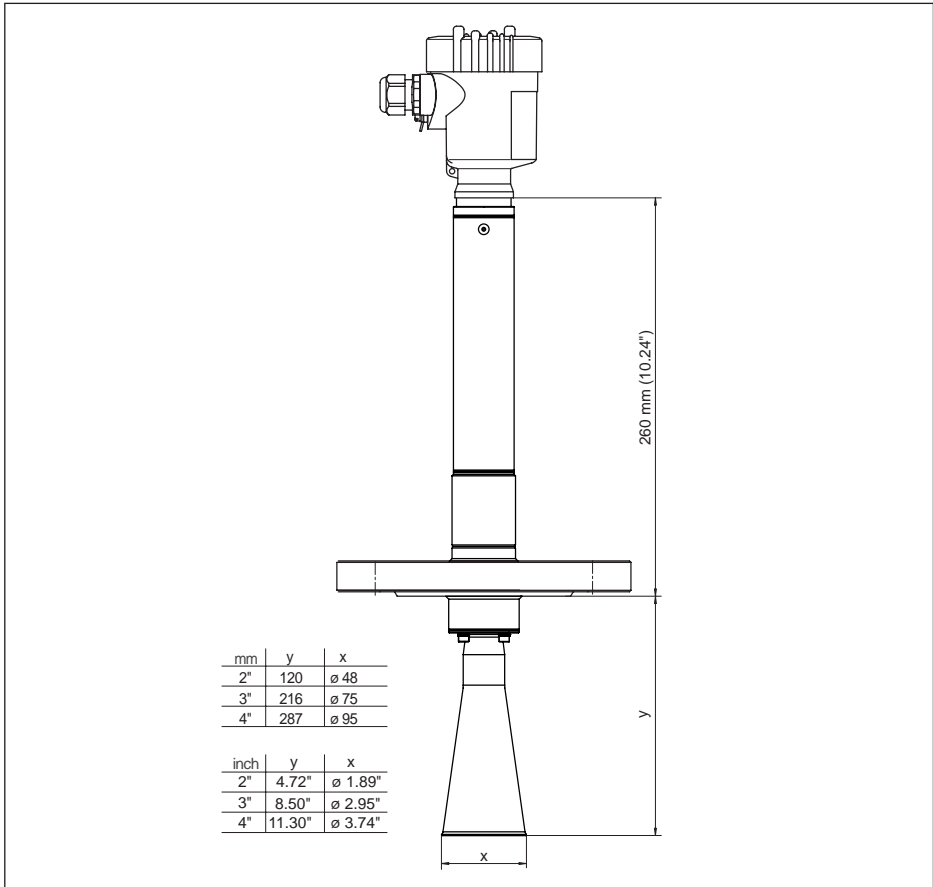
Figura 67: VEGAPULS 62, antenna a cono in esecuzione a flangia con pezzo intermedio per alte temperature fino a 450 °C
