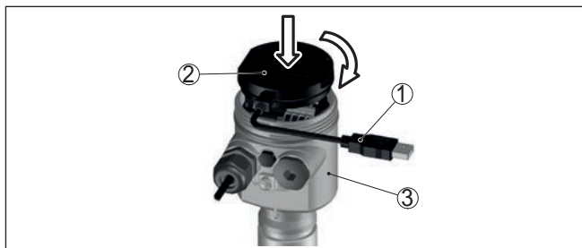
Figura 39: Collegamento diretto del PC al sensore via adattatore d'interfaccia
