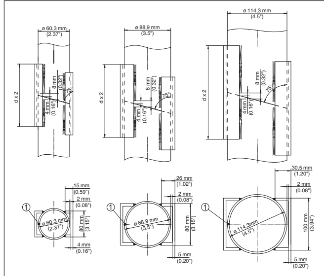
Figura 19: Saldatura per prolungamento del tubo di calma per diversi esempi di diametro
