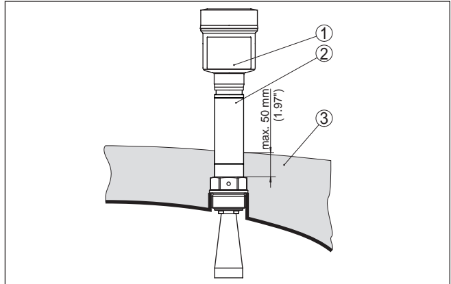
Figura 17: Montaggio dell'apparecchio su un serbatoio isolato.
