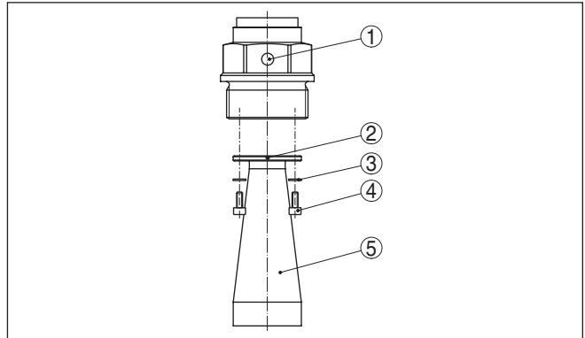
Figura 2: Smontaggio dell'antenna a cono
