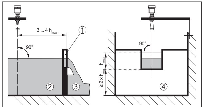
Figura 21: Misura di portata con stramazzo rettangolare: d_{min} = distanza minima del sensore (vedi capitolo "Dati tecnici"); h_{max} = max. riempimento dello stramazzo rettangolare
