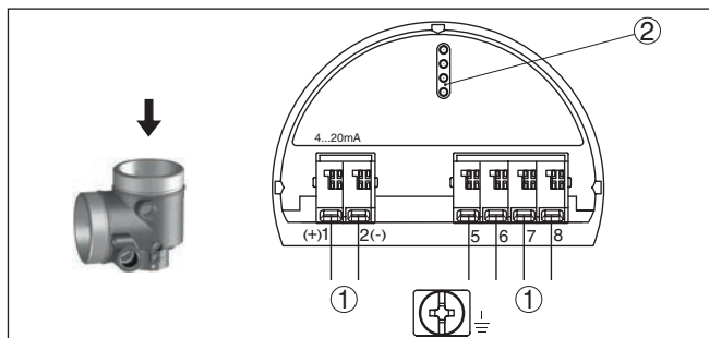
Figura 25: Vano dell'elettronica - custodia a due camere
