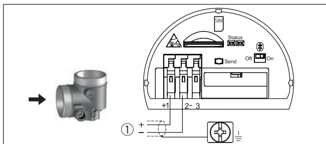
Figura 27: Vano di connessione - modulo radio PLICSMOBILE 81
