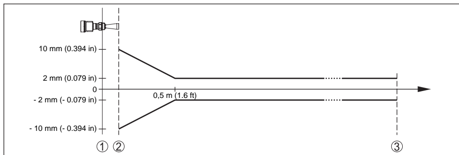
Figura 58: Scostamento di misura sotto condizioni di riferimento
