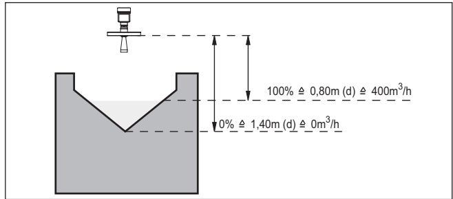
Fig. 21: Réglage de la mesure de débit dans un déversoir triangulaire
