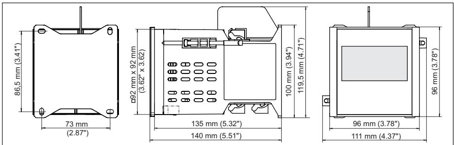
Fig. 23: Encombrement VEGAMET 391
