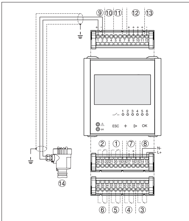
Fig. 5: Schéma de raccordement avec capteur bifilaire
