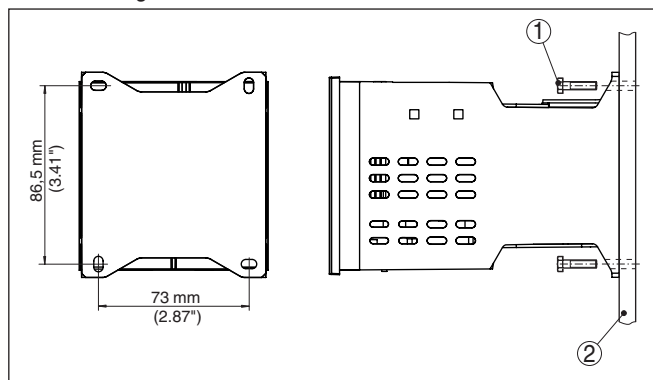
Fig. 3: Fixation par vis
