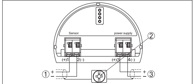
Fig. 13: Esquema de conexión VEGAWELL 52 para sensores 4 ... 20 mA
