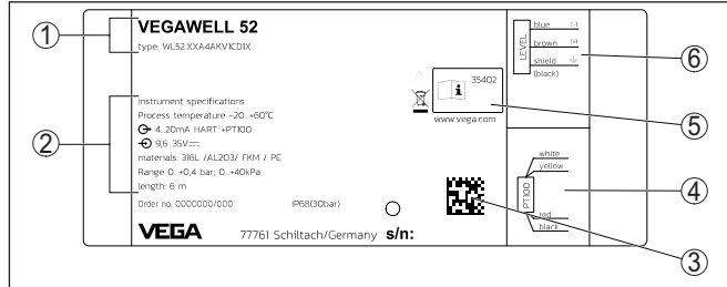
Fig. 2: Estructura de la placa de tipos (ejemplo)
