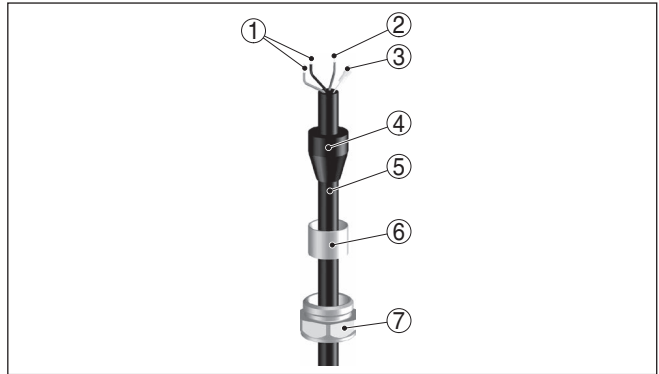
Fig. 15: Montaje del sello del cable
