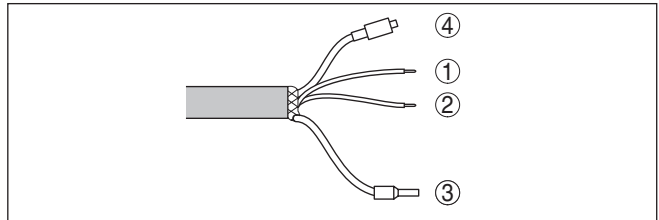
Fig. 10: Ocupación de conductores del cable portador
