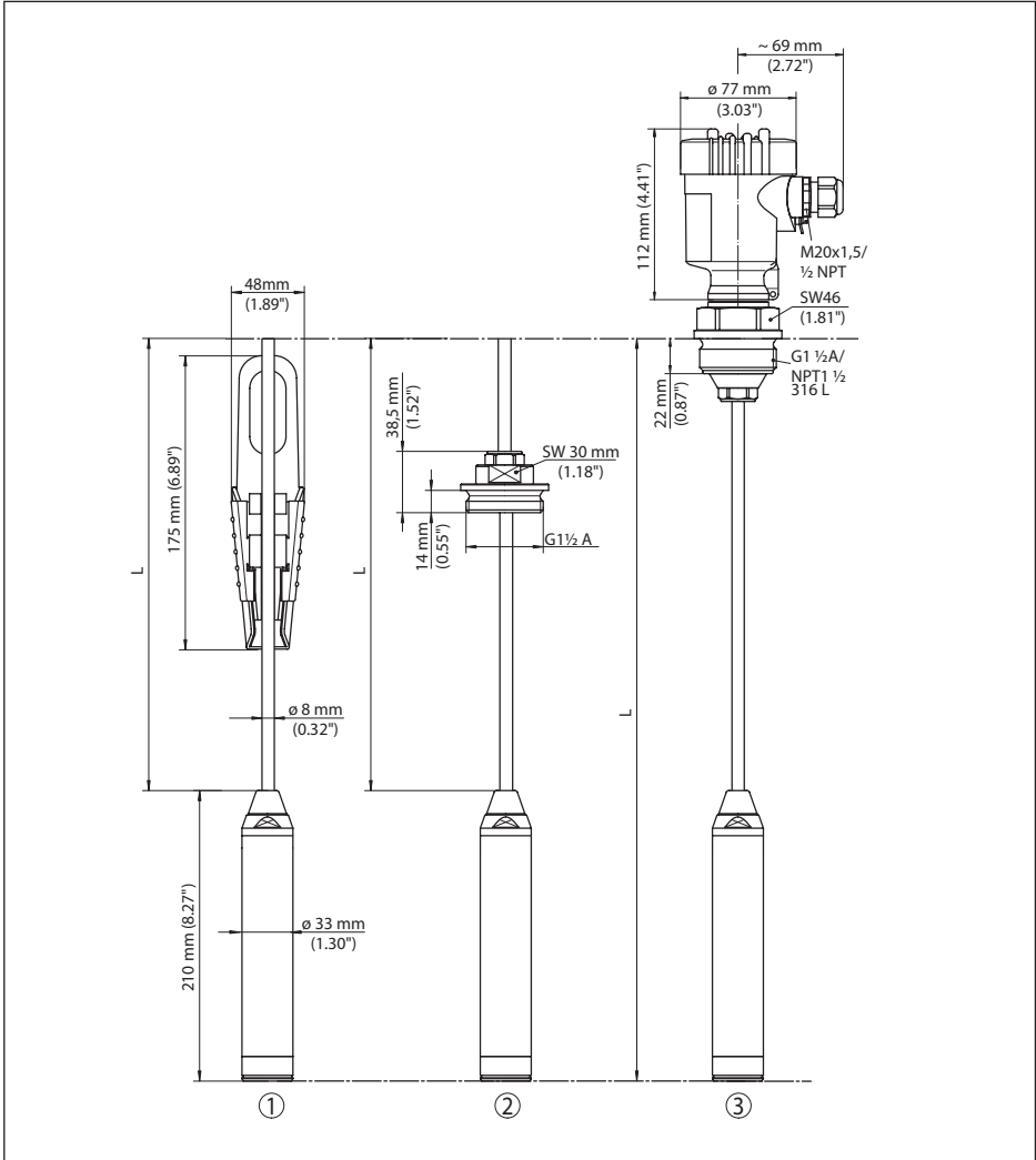
Fig. 17: VEGAWELL 52, con sensor de valores medidos de titanio 33 mm
