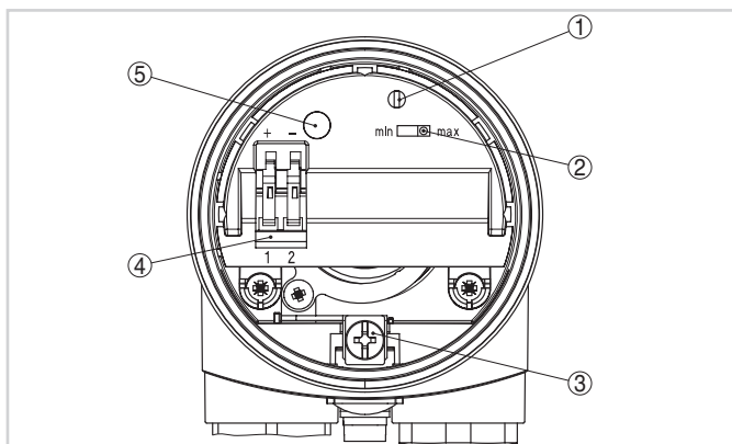
Compartiment électronique et de raccordement - sortie bifilaire
