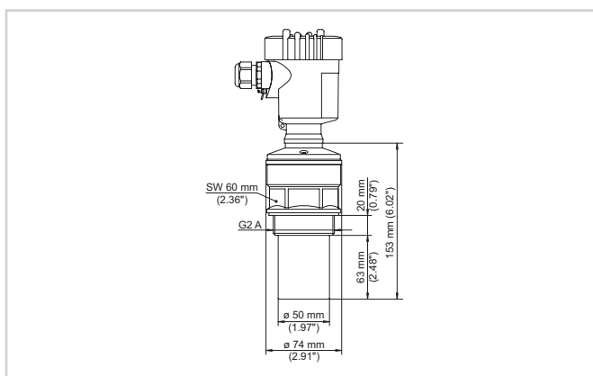
Dimensões VEGASON 62
