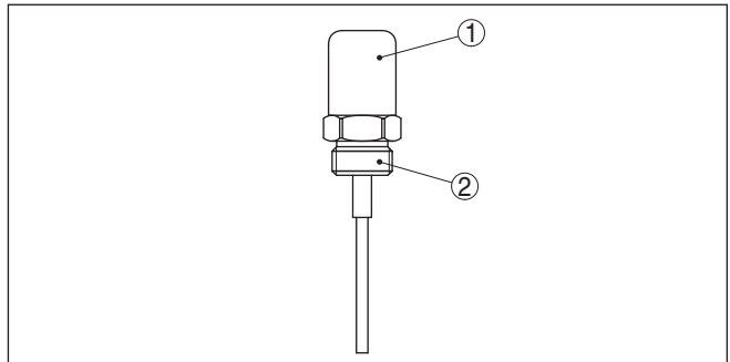
Fig. 1: Sonde de mesure résistive à tige EL 8
