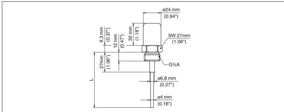
Fig. 5: Sonde de mesure résistive à tige EL 8
