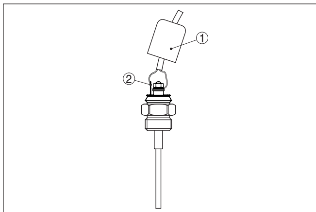
Fig. 4: Connexion à la masse (en option)
