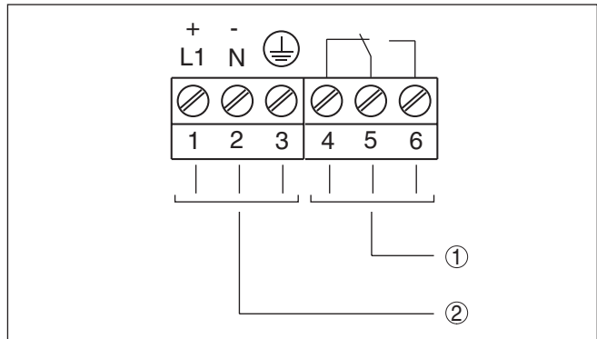
Fig. 4: Électronique avec sortie relais
