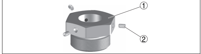
Fig. 1: Racor de fijación ARV-WE63.1 - sin presión
