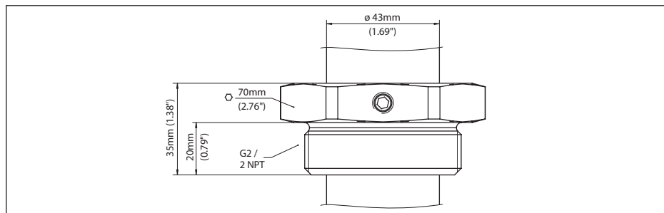
Fig. 2: Racor de retención ARV-WE63.1 sin presión para VEGAWAVE 63
