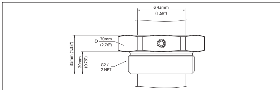
Fig. 2: Raccord d'arrêt ARV-WE63.1 sans pression pour VEGAWAVE 63
