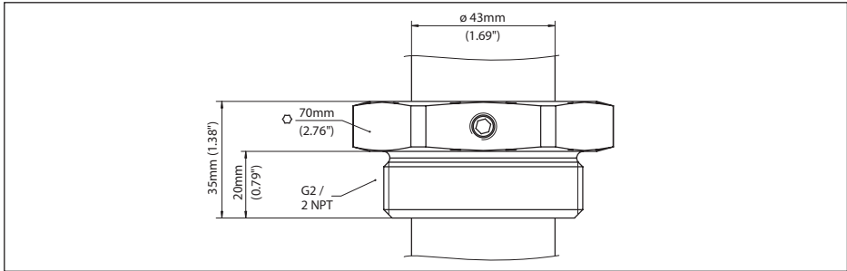
Res. 2: Basıncısız VEGAWAVE 63 için durdurma dişlisi ARV-WE63.1
