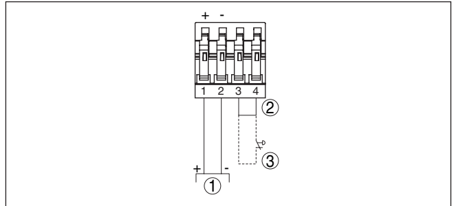
Fig. 11: Esquema de conexión - Tecla externa de simulación
