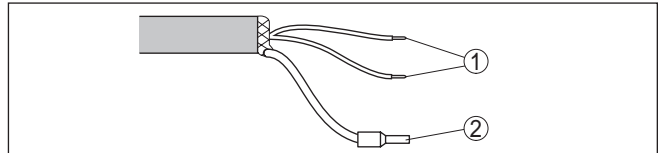
Fig. 12: Ocupación de conductores del cable de conexión
