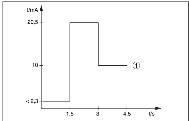
Abb. 13: Anlaufverhalten
