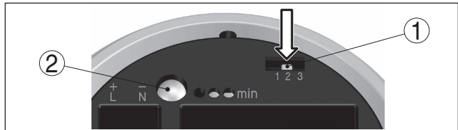
Abb. 19: Kompensationstaster
