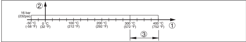
Abb. 20: Prozesstemperatur - Prozessdruck
