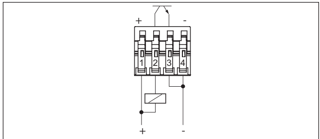
Rys. 12: Podłączenie NPN
