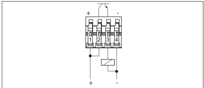
Rys. 13: Podłączenie PNP
