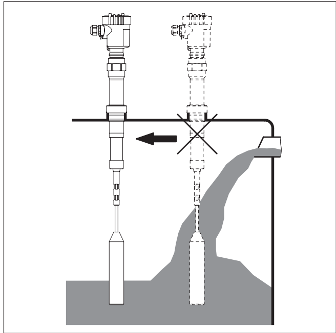
Rys. 5: Wpływające medium
