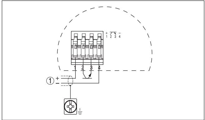
Rys. 11: Schemat przyłączy
