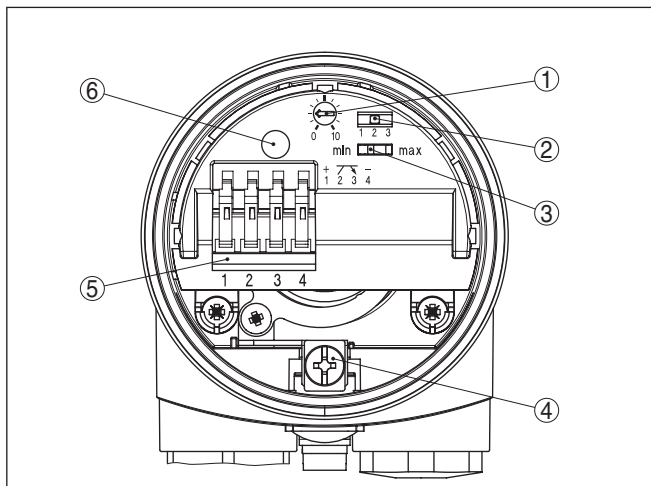
Fig. 10: Compartimento do sistema eletrônico e de conexão
