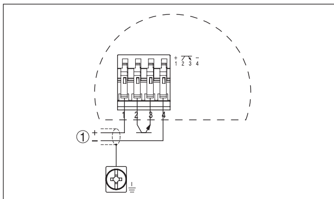
Fig. 11: Esquema de ligações
