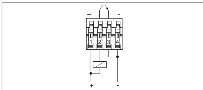
Fig. 12: Comportamento NPN
