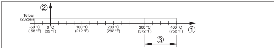
Fig. 20: Temperatura do processo - Pressão do processo
