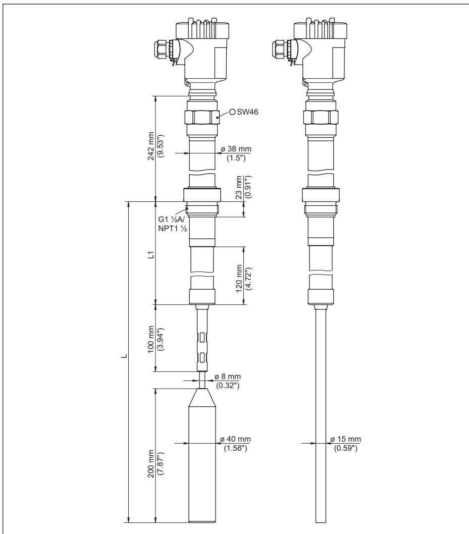
Fig. 23: VEGACAP 67, modelo com rosca G1 1/2 (ISO 228 T1) e 1 1/2 NPT, -50 ... +300 °C (-58 ... +572 °F)
