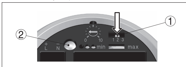
Fig. 18: Botão de compensação
