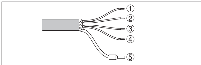
Fig. 14: Atribuição dos fios. Os números dos fios correspondem aos terminais do aparelho.
