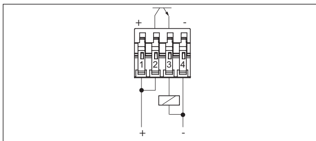
Fig. 13: Comportamento PNP
