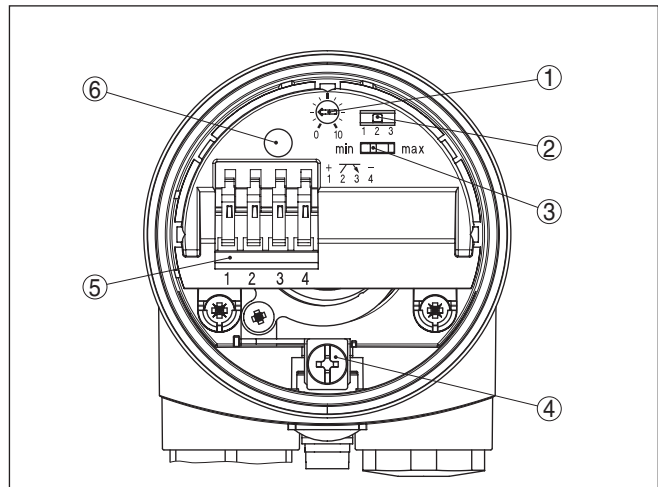
Fig. 15: Sistema eletrônico - saída do transistor
