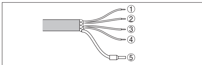
Fig. 14: Affectation des conducteurs du câble de raccordement. Les numéros des conducteurs correspondent aux bornes de raccordement de l'appareil.
