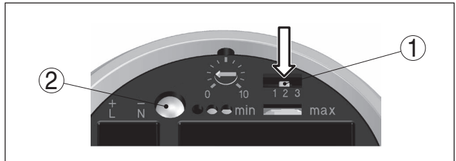
Fig. 19: Touche de compensation
