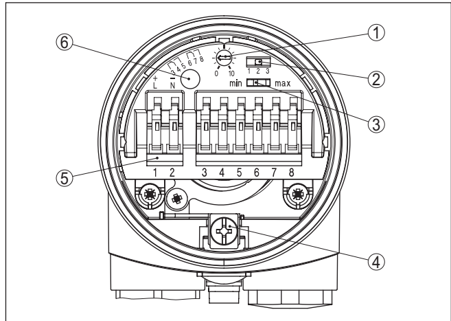
Fig. 12: Sistema eletrônico - saída do relé
