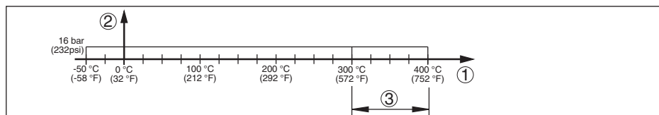
Fig. 17: Temperatura do processo - Pressão do processo
