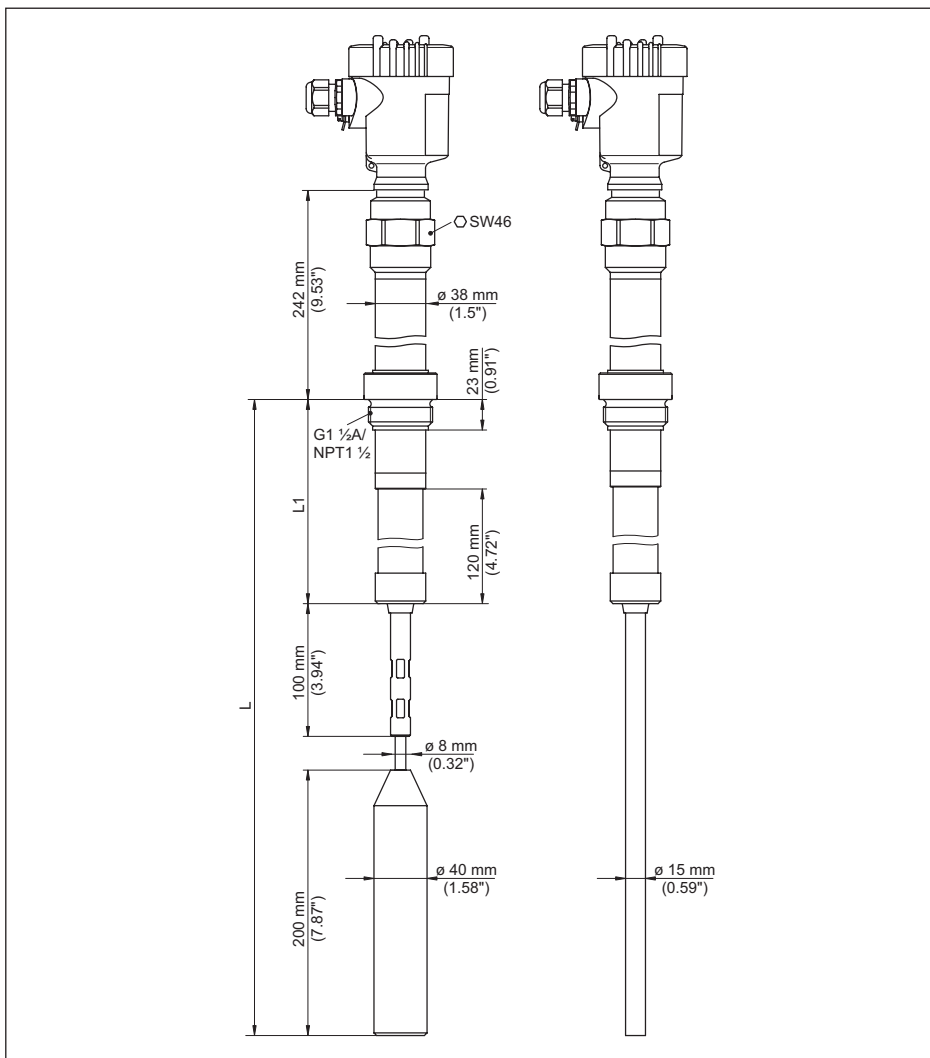
Fig. 19: VEGACAP 67, modelo com rosca G1½ (ISO 228 T1) e 1½ NPT, -50 ... +300 °C (-58 ... +572 °F)
