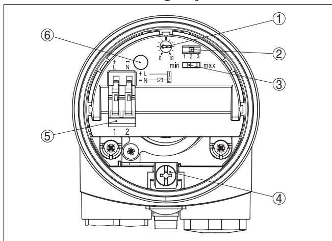
Fig. 12: Sistema eletrônico - interruptor sem contato
