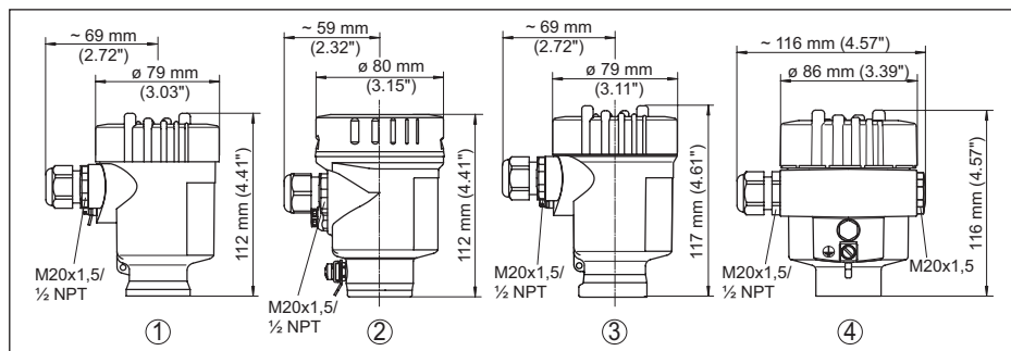
Fig. 18: Modelos da caixa
