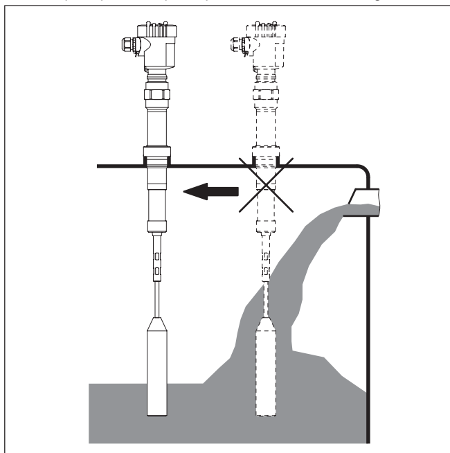
Fig. 5: Fluxo de entrada do produto
