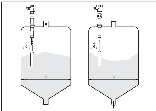
Fig. 6: Enchimento e esvaziamento no centro
