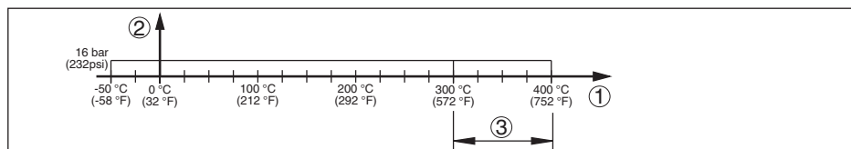
Fig. 17: Temperatura do processo - Pressão do processo
