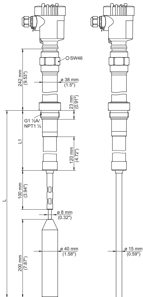
Fig. 19: VEGACAP 67, versión roscada G1½ (ISO 228 T1) y 1½ NPT, -50 ... +300 °C (-58 ... +572 °F)
