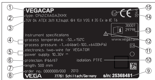
Fig. 2: Estructura de la placa de tipos (ejemplo)
