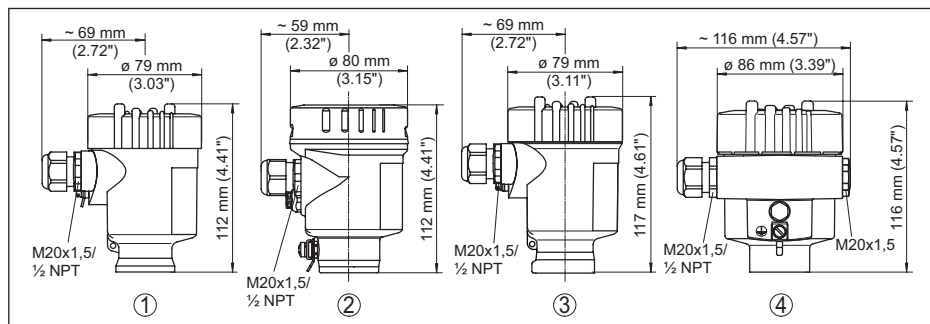
Fig. 18: Versiones de carcasas
