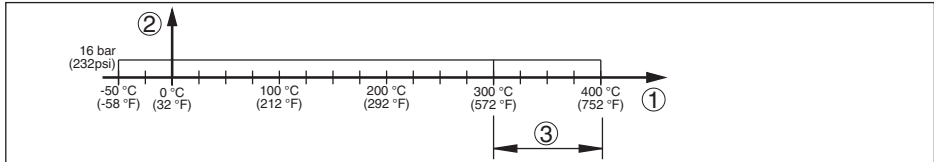
Fig. 17: Presión proceso - Temperatura de proceso
