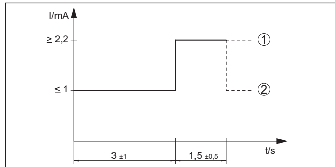
Fig. 14: Diagrama secuencial de la prueba de funcionamiento - función de conmutación en correspondencia con el estado de cobertura y selección de curva característica (ver tabla de funciones)
