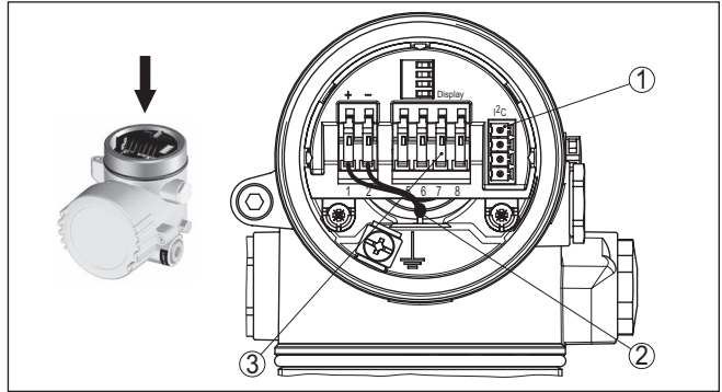
Res. 16: Elektronik bölümü - İki hücreli gövde
