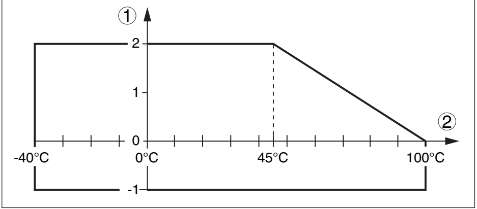
Res. 29: Proses basıncı - Proses sıcaklığı (PTFE flanş)
