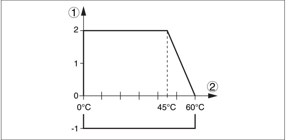
Res. 30: Proses basıncı - Proses sıcaklığı (PP flanş)
