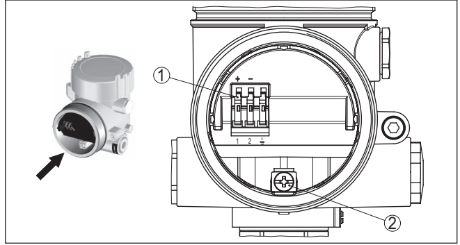
Res. 17: Ex d ia iki hücreli gövde - bağlantı bölgesi
