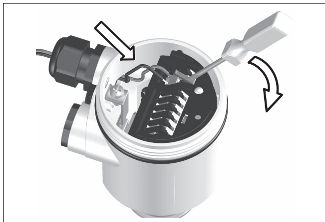
Rys. 6: Czynności przy podłączeniu 5 i 6
