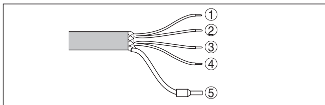
Rys. 12: Konfiguracja żył kabla podłączeniowego. Numery żył odpowiadają numerom zacisków przyrządu.
