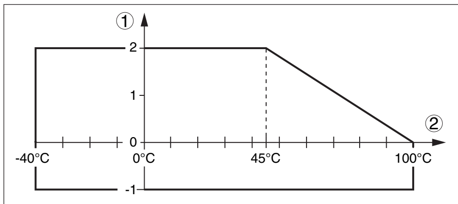
Rys. 17: Ciśnienie i temperatura technologiczna (kolnierz z PTFE)
