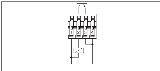
Rys. 10: Podłączenie NPN
