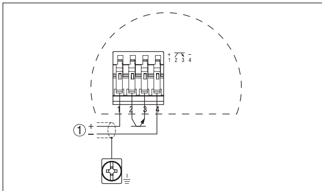
Rys. 9: Schemat przyłączy
