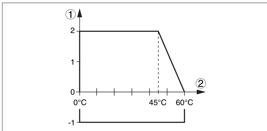
Rys. 18: Ciśnienie i temperatura technologiczna (kolnierz z PP)
