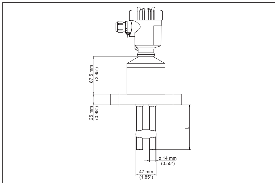
Rys. 21: VEGACAP 69
