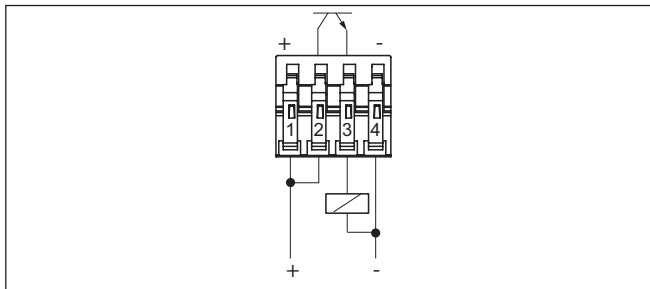
Rys. 11: Podłączenie PNP
