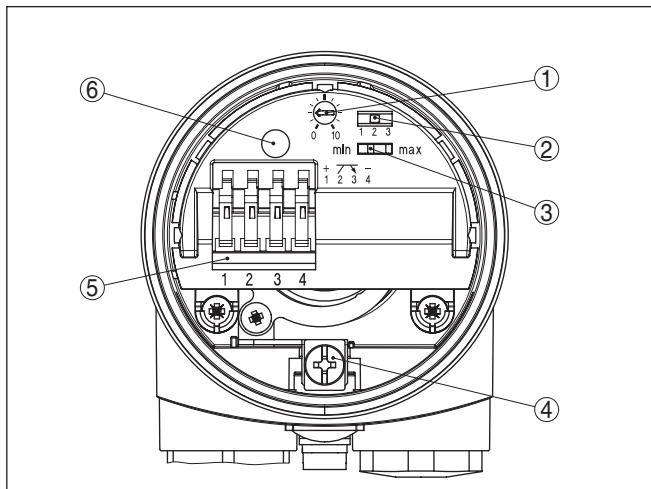
Rys. 13: Moduł elektroniczny - wyjście tranzystorowe
