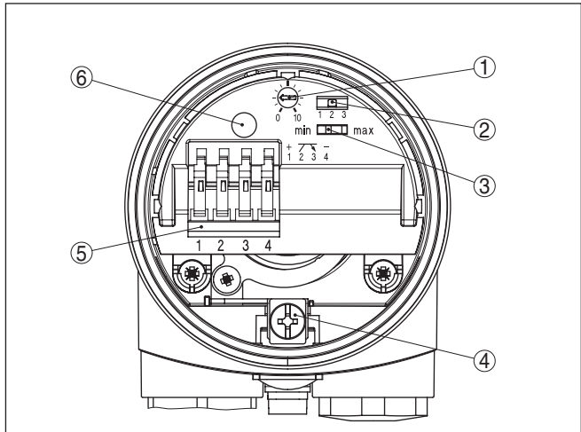
Rys. 8: Komora układu elektronicznego i przyłączy
