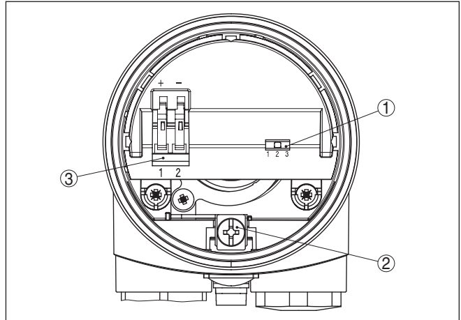
Rys. 13: Wyświetlacz i elementy obsługowe - moduł elektroniczny
