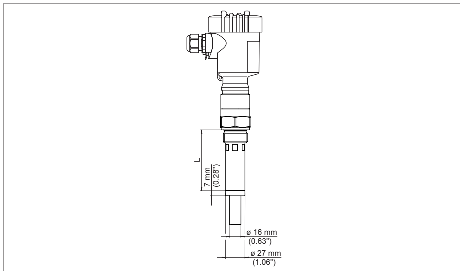
Rys. 20: VEGACAL 66, rura ekranująca np. z powodu intensywnego wydzielenia skroplin
