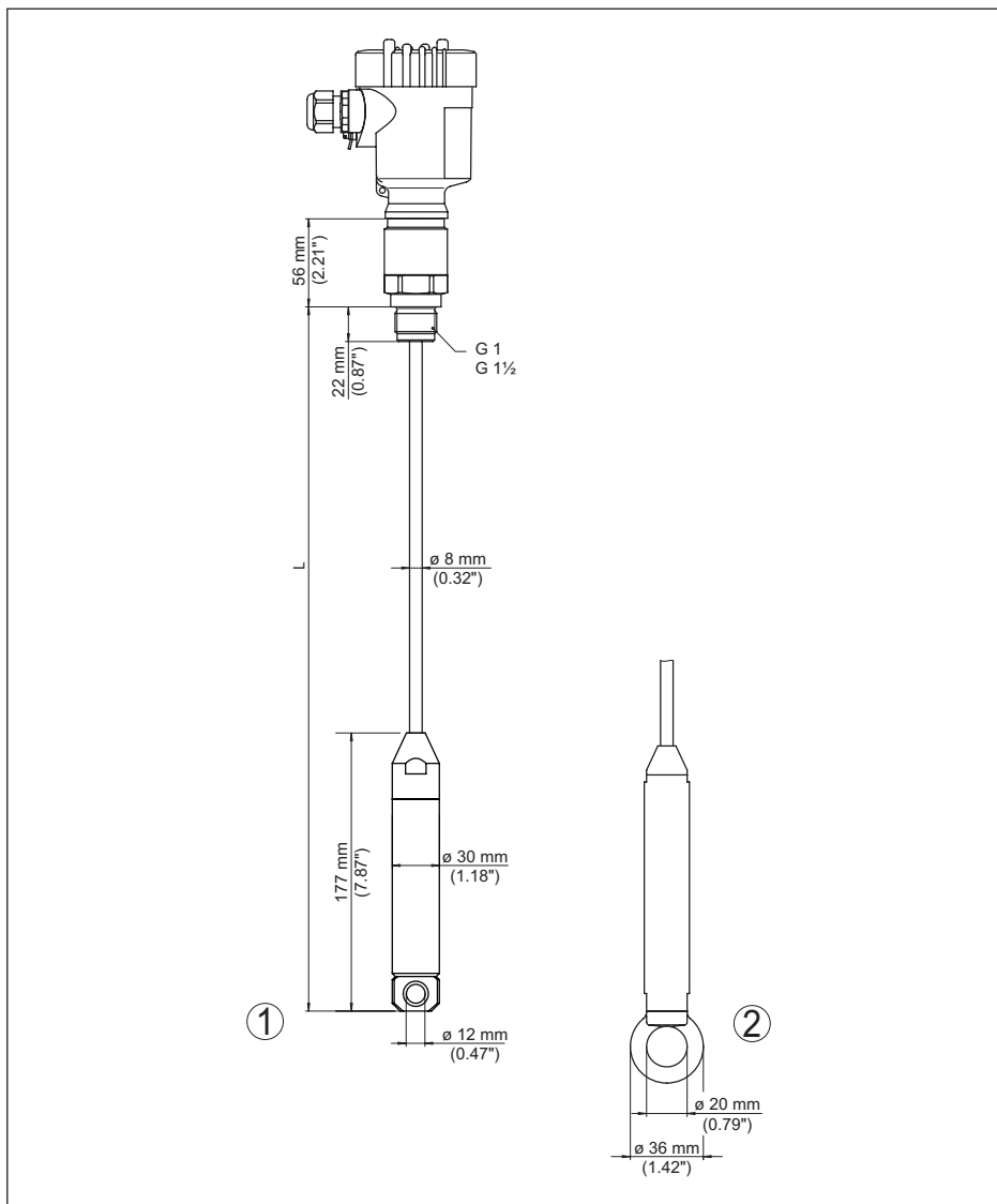
Rys. 19: VEGACAL 66, wersja z gwintem G1 (ISO 228 T1)
