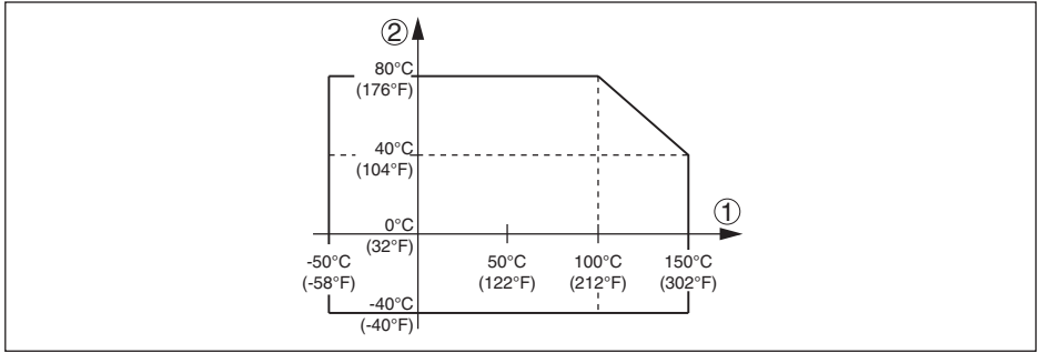
Res. 15: Ortamdaki maddenin sıcaklığı - Proses sıcaklığı
