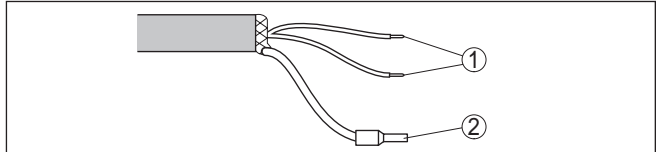
Res. 12: Tel atama bağlantı kablosu
