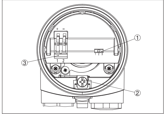
Res. 13: Gösterge ve ayar elemanları - Elektronik modül
