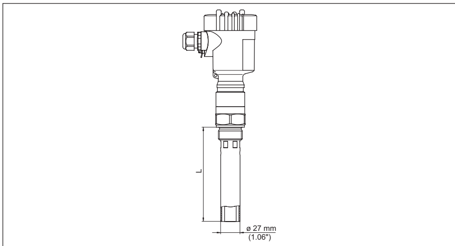
Fig. 22: VEGACAL 62, tube de référence, p. ex. si faible constante diélectrique ou pour linéarisation
