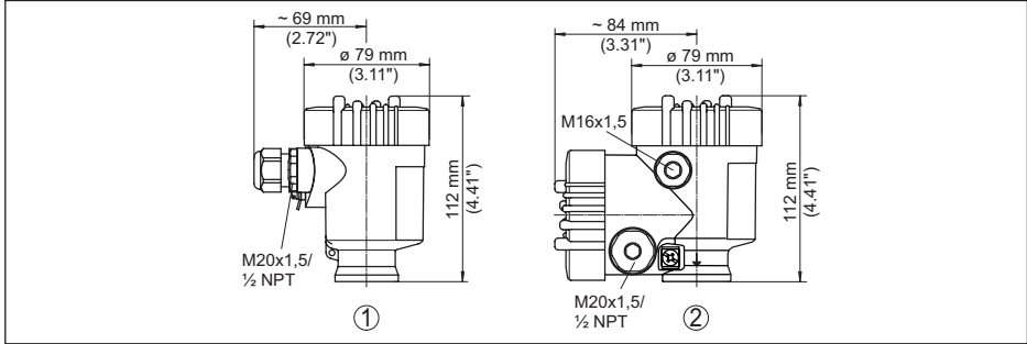
Res. 31: IP66/IP67 koruma tipli gövde modelleri (Entegre gösterge ve ayar modülü gövde yüksekliğini 9 mm/0.35 in artırır.)
