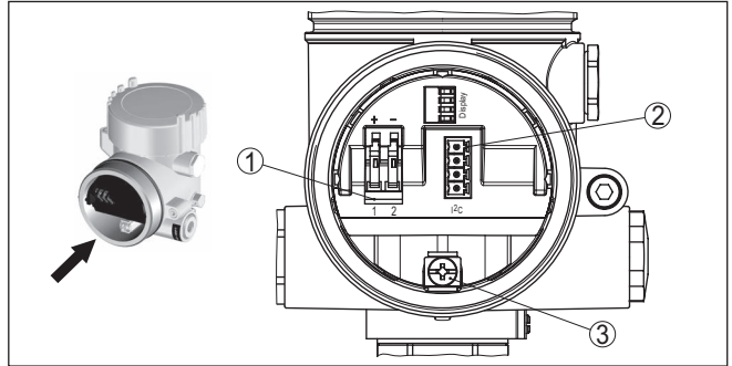
Res. 14: İki hücreli gövde - bağlantı bölmesi
