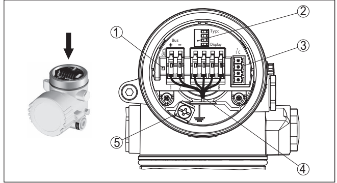
Res. 13: Elektronik bölmesi - iki hücreli gövde
