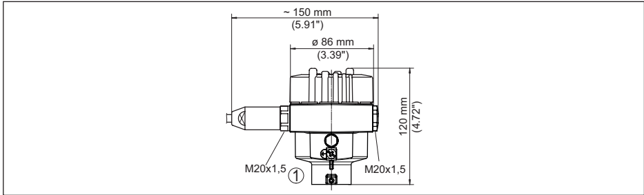
Res. 32: Koruma sınıfı IP66/IP68 (1 bar) olan gövde modelleri; (entegre gösterge ve ayar modülü gövde yüksekliğini 18 mm/0.71 in kadar artırır)
