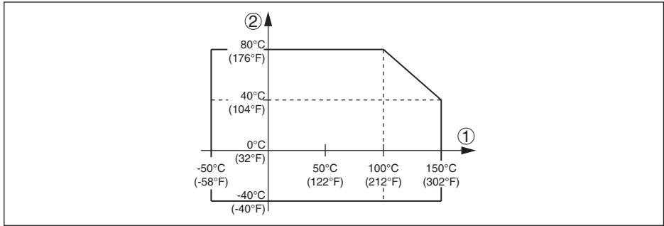
Res. 28: Ortamdaki maddenin sıcaklığı - Proses sıcaklığı
