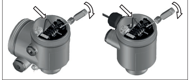
Res. 8: Bağlantı prosedürü 6 ve 7
