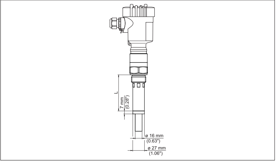
Res. 34: VEGACAL 66, ör. şiddetli yağuşum olmasına karşı yalıtımlı boru
