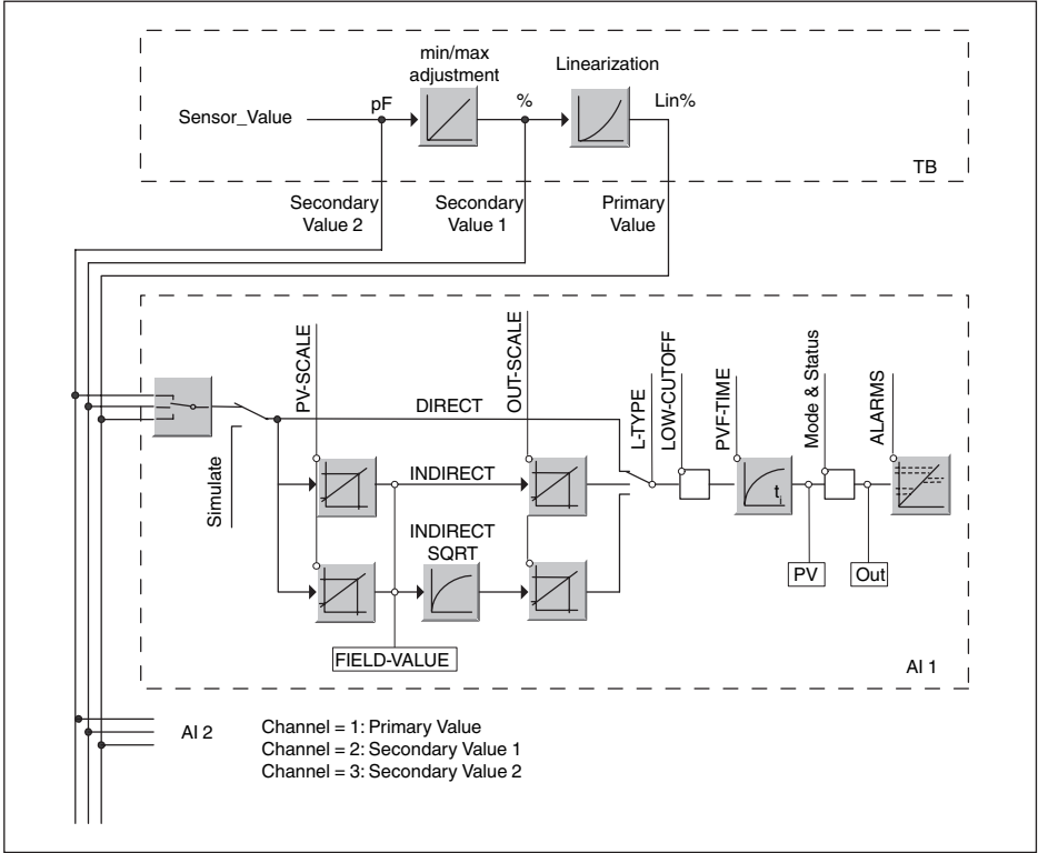
Res. 29: VEGACAL 66 ölçüm değerli işlem
