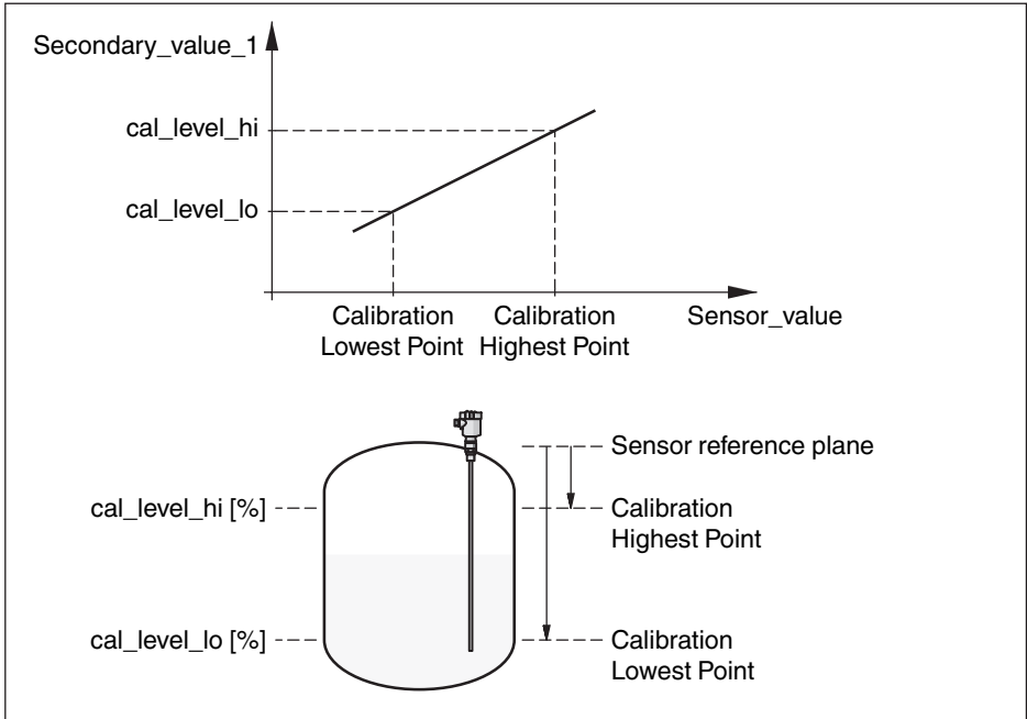
Res. 30: Ayar VEGACAL 66
