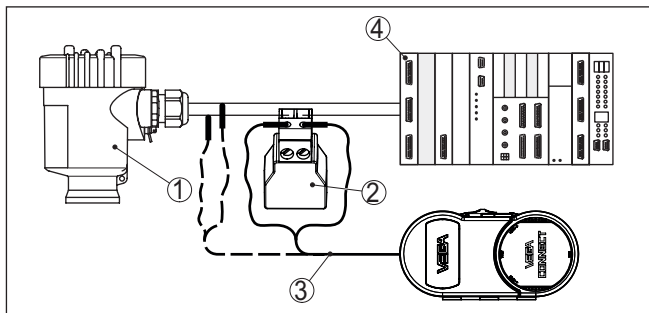
Rys. 25: Podłączenie PC przez HART z przewodem sygnałowym
