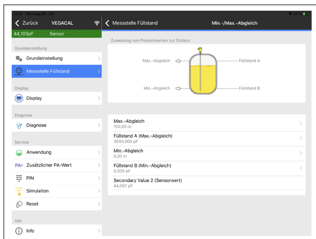
Rys. 28: Przykładowy obraz aplikacji rozruchu - dostrojenie przetwornika pomiarowego
