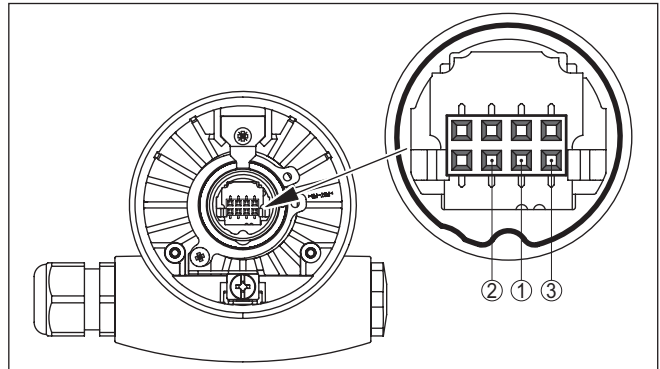
Rys. 29: Sprawdzenie rezystancji wewnątrz sondy pomiarowej
