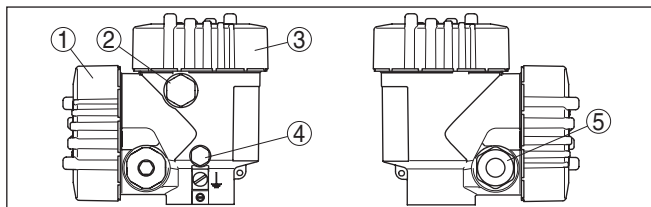
Rys. 12: Obudowa dwukomorowa
