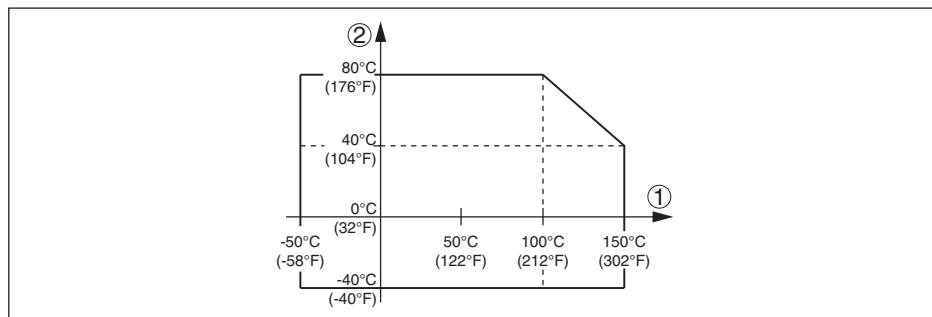
Rys. 30: Temperatura otoczenia - temperatura procesu technologicznego
