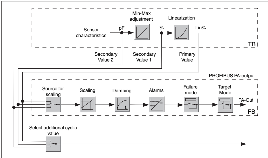
Fig. 29: VEGACAL 64: blokschema met AI (PA-OUT)-waarde en extra cyclische waarde
