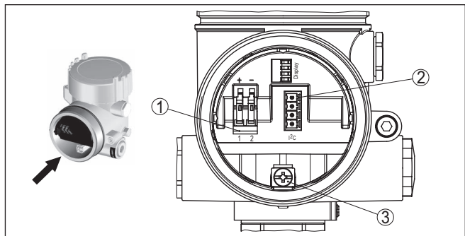
Fig. 14: Aansluitruimte - tweekamerbehuizing
