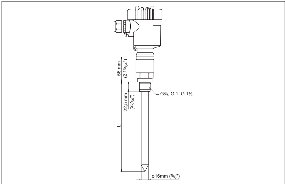
Fig. 34: VEGACAL 64 - versión roscada G1(ISO 228 T1)
