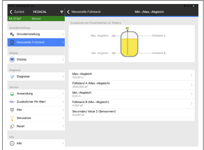
Fig. 28: Exemplo de uma vista do App - colocação em funcionamento - calibração do sensor
