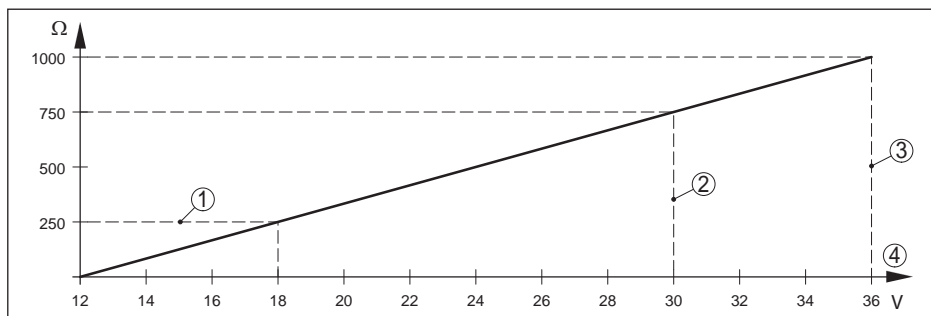
Fig. 31: Diagrama de tensão
