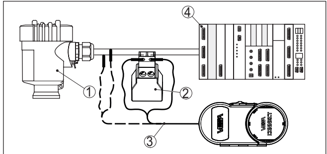
Fig. 25: Conexão do PC à linha de sinais via HART
