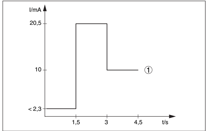
Fig. 13: Comportamiento de arranque
