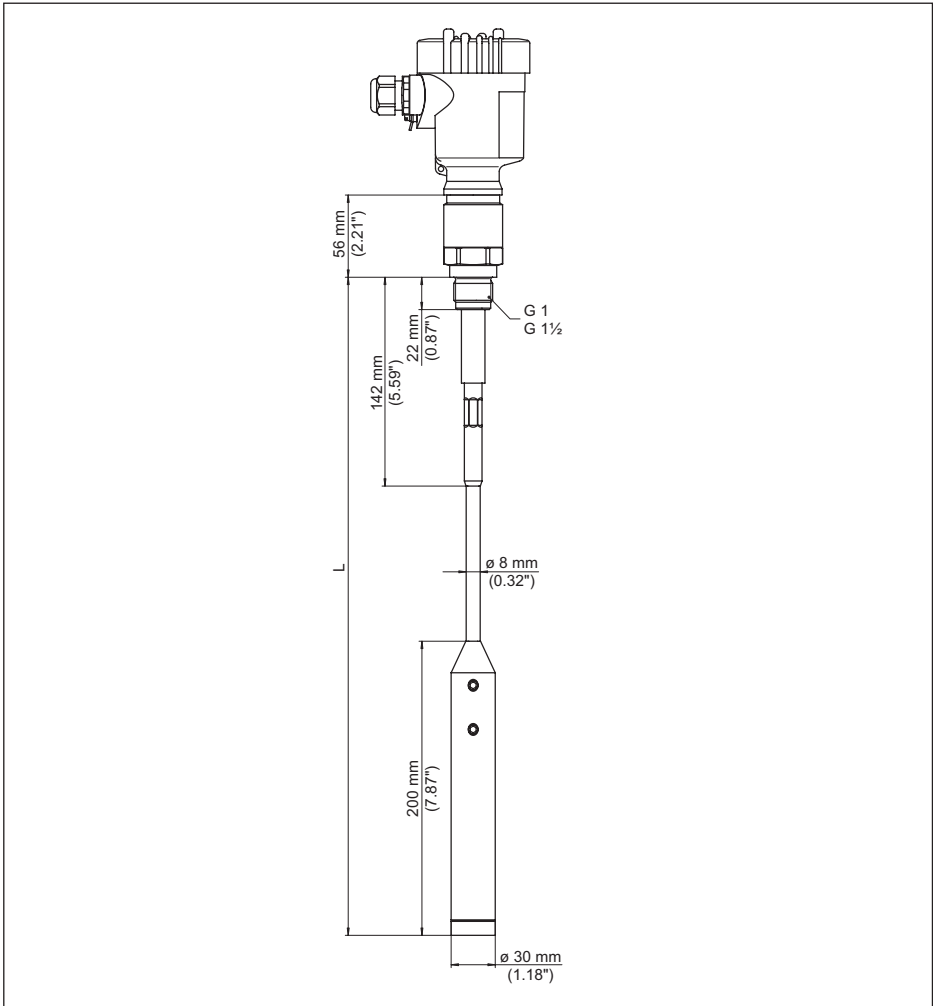
Fig. 25: VEGACAP 65, versión de cable con \varnothing 8 mm (0.315 in), versión de rosca G1 (ISO 228 T1)
