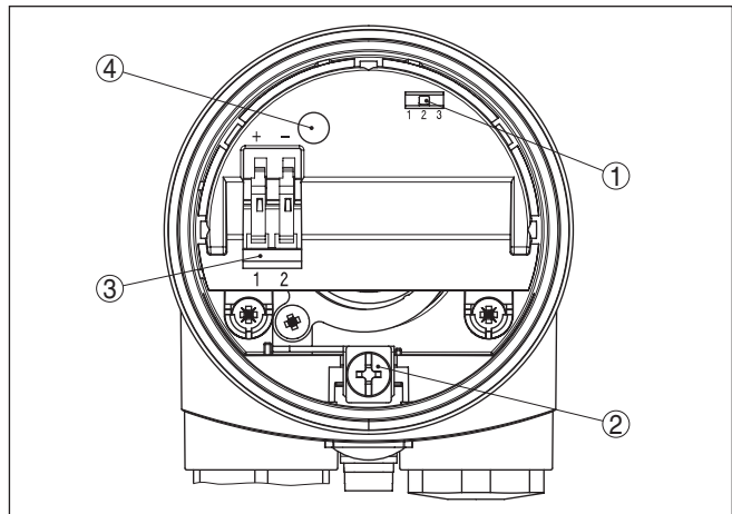
Fig. 14: Módulo electrónico - Salida de dos conductores
