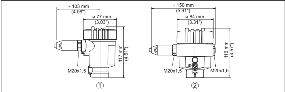
Abb. 23: Gehäuseausführungen in Schutzart IP66/IP68 (1 bar)
