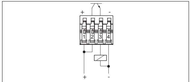
Abb. 13: PNP-Verhalten
