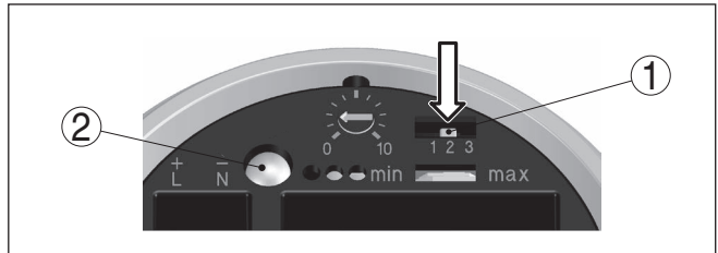
Abb. 20: Kompensationstaster
