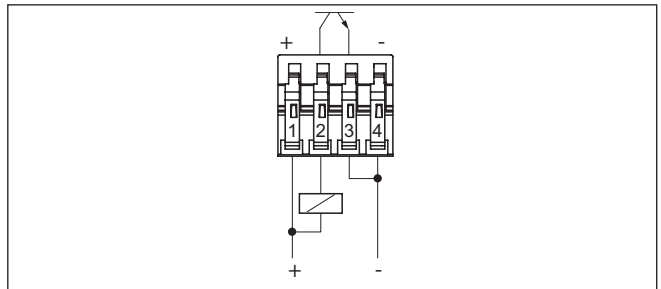
Abb. 12: NPN-Verhalten
