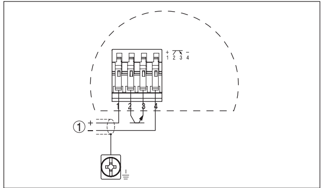
Abb. 11: Anschlussplan
