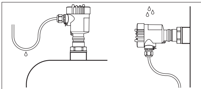
Fig. 4: Medidas para evitar a entrada de umidade
