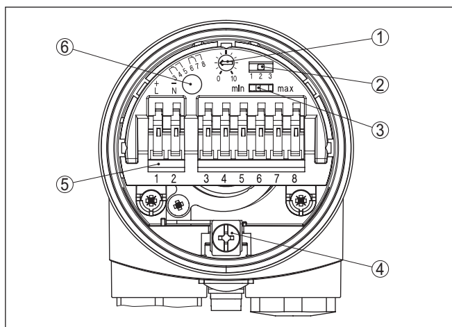
Figura 11: Unità elettronica con uscita a relé
