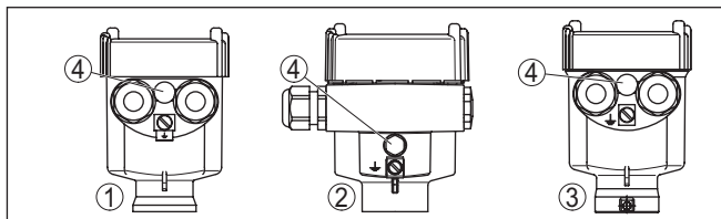
Figura 8: Differenti materiali - custodia ad una camera
