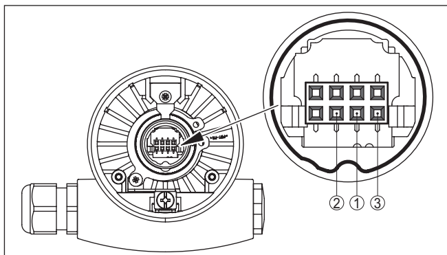
Figura 12: Controllare la resistenza all'interno della sonda di misura
