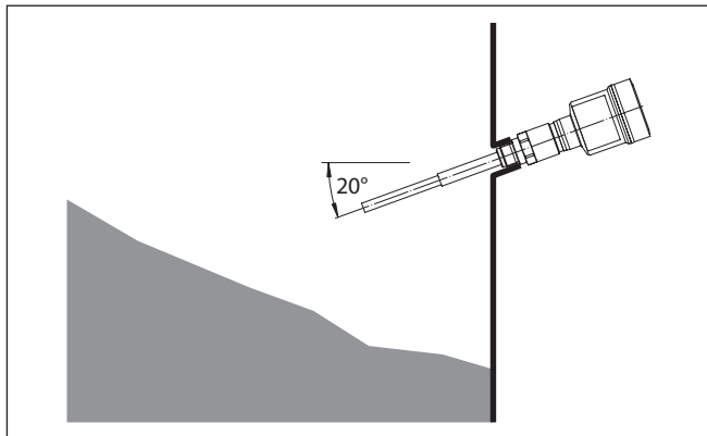
Figura 6: Montaggio orizzontale
