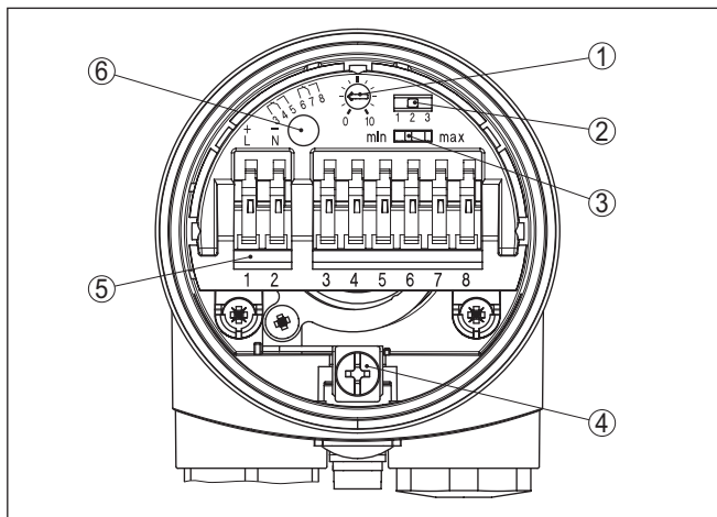
Figura 9: Vano dell'elettronica e di connessione
