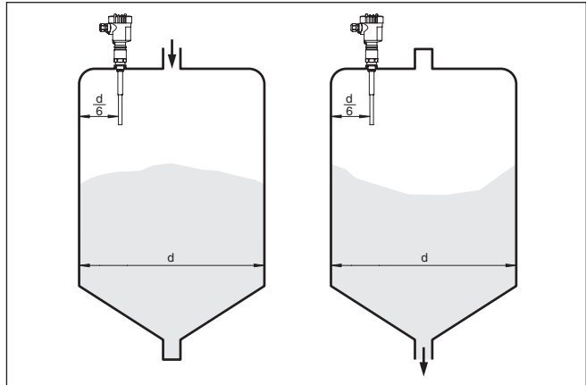
Fig. 7: Enchimento e esvaziamento no centro
