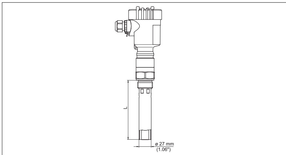
Fig. 27: VEGACAP 62, tubo envoltório, por exemplo, no caso de baixo coeficiente dielétrico ou para a linearização
