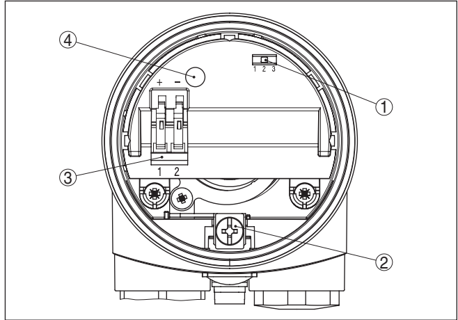
Fig. 11: Compartimento do sistema eletrônico e de conexão
