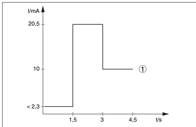
Fig. 14: Comportamento de partida
