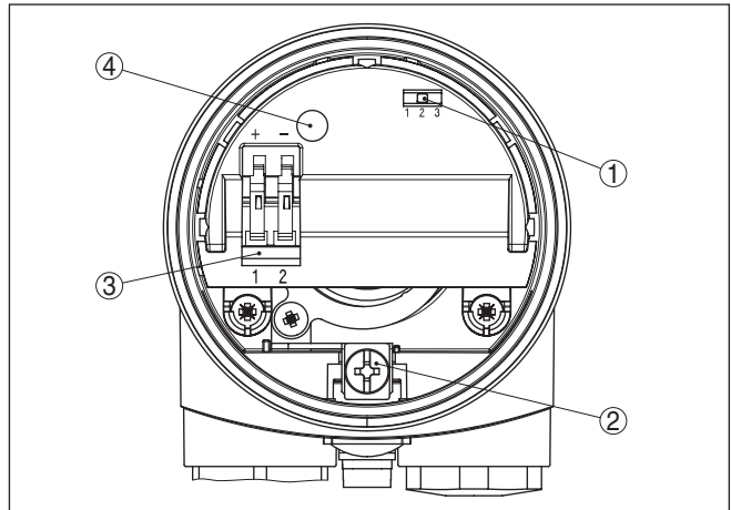
Fig. 15: Sistema eletrônico - Saída de dois condutores
