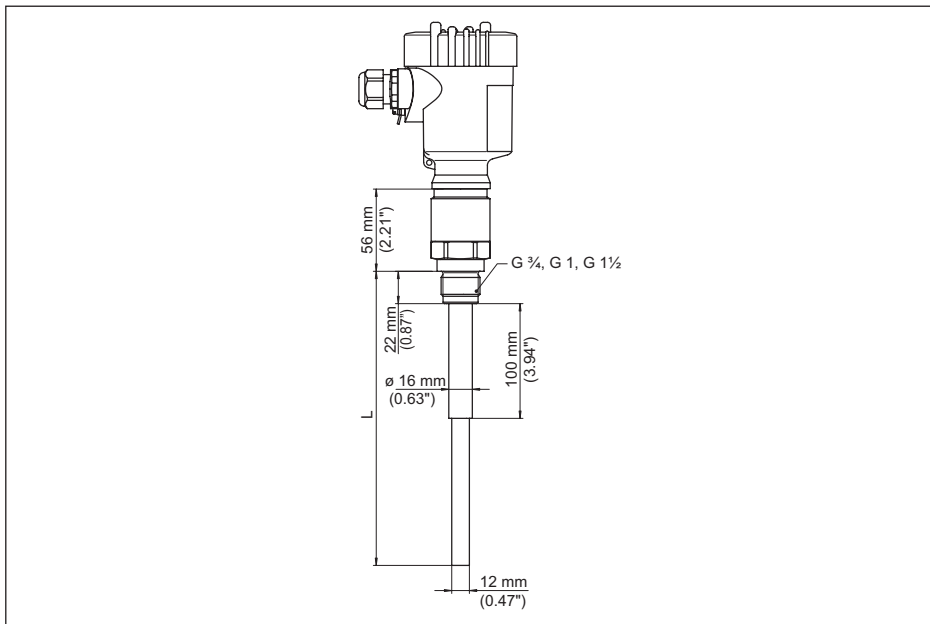
Fig. 24: VEGACAP 62, modelo com rosca G1 (ISO 228 T1)
