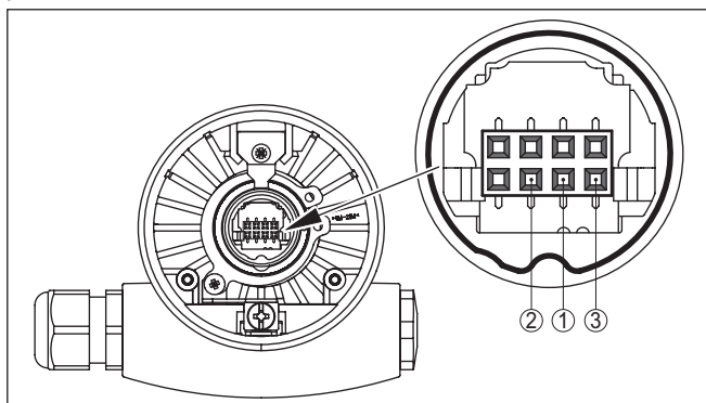
Fig. 17: Verificar a resistência dentro da sonda de medição
