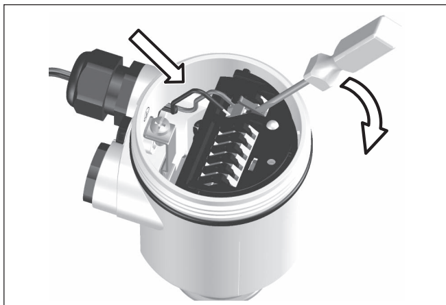
Rys. 9: Czynności przy podłączaniu 5 i 6
