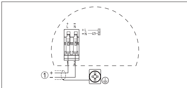
Rys. 12: Schemat przyłączy
