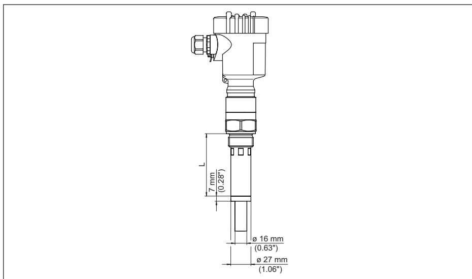
Rys. 22: VEGACAP 62, rura ekranująca np. z powodu intensywnego wydzielania skroplin
