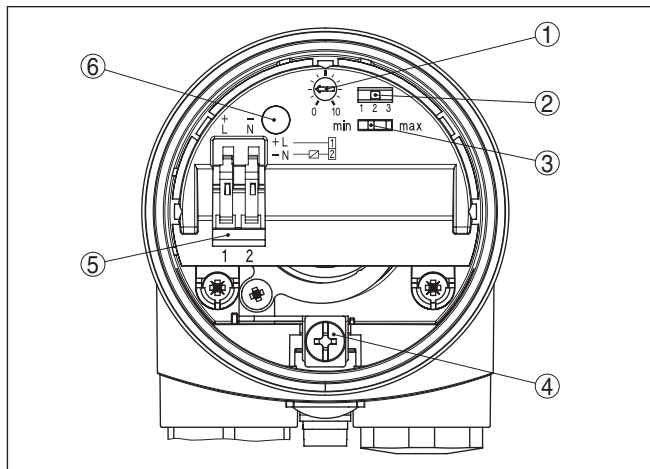
Rys. 13: Moduł elektroniczny - przełącznik bezstykowy
