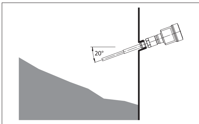
Fig. 6: Montagem horizontal
