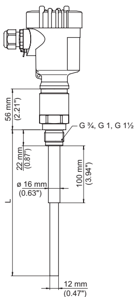
Fig. 20: VEGACAP 62, modelo com rosca G1 (ISO 228 T1)
