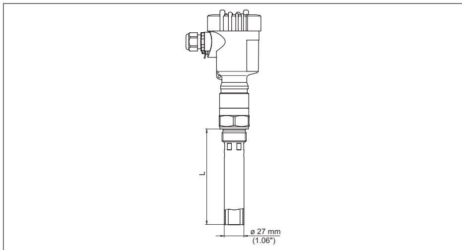
Fig. 23: VEGACAP 62, tubo envoltório, por exemplo, no caso de baixo coeficiente dielétrico ou para a linearização
