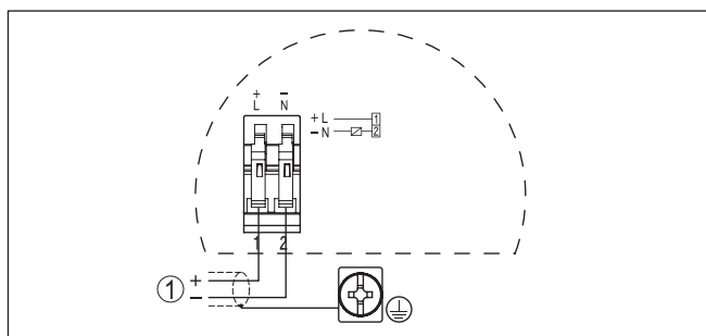
Fig. 12: Esquema de ligações
