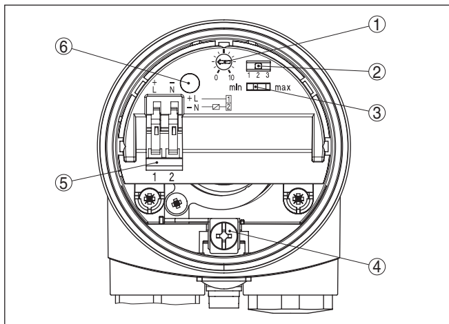
Fig. 11: Compartimento do sistema eletrônico e de conexão
