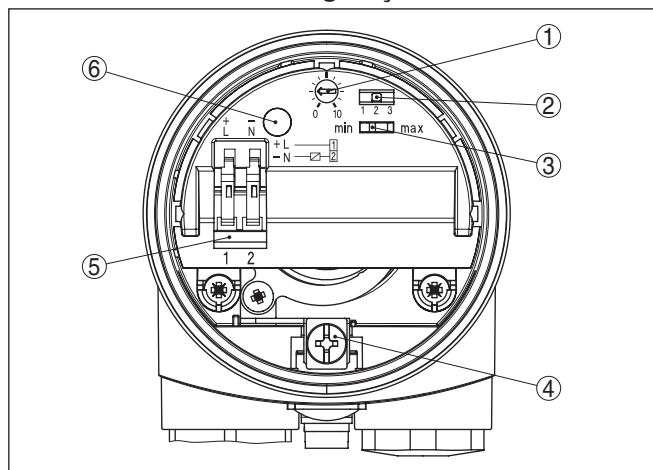
Fig. 13: Sistema eletrônico - interruptor sem contato
