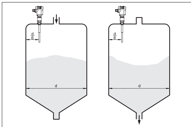
Fig. 7: Enchimento e esvaziamento no centro
