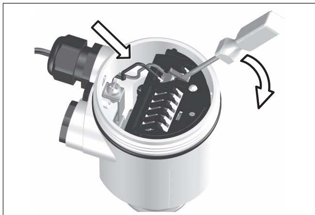
Fig. 9: Passos 5 e 6 do procedimento de conexão
