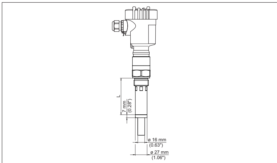
Fig. 22: VEGACAP 62, tubo de blindagem, por exemplo, contra forte condensação
