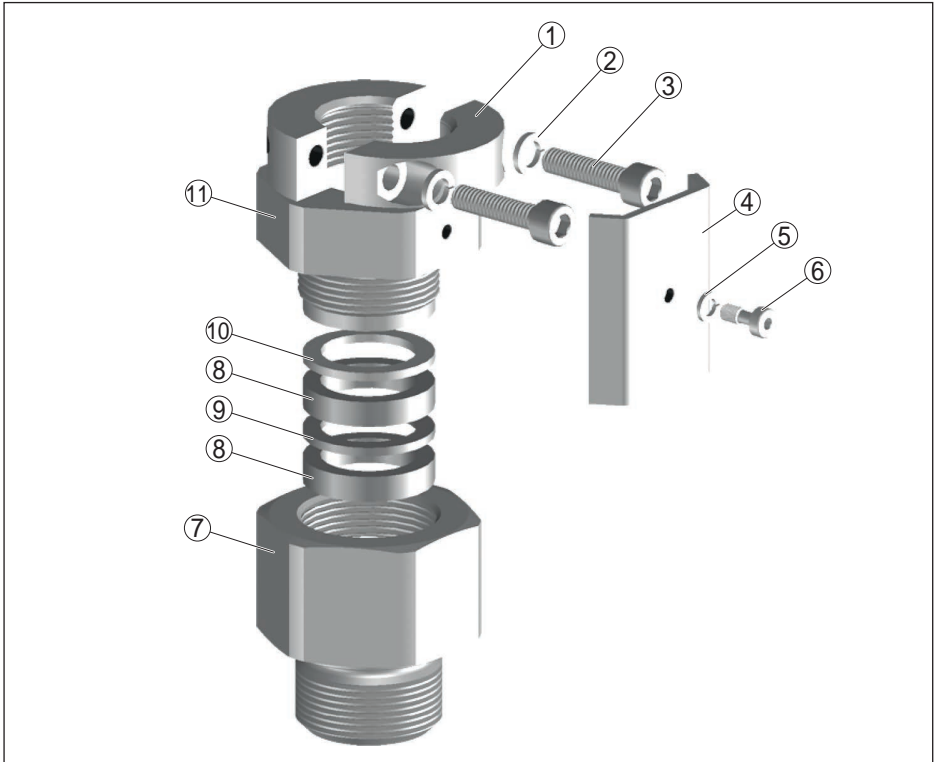
Fig. 1: Raccord d'arrêt ARV-VB63.2 - jusqu'à 16 bar (232 psig)
