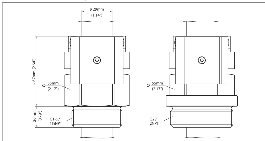
Fig. 2: Raccord d'arrêt ARV-VB63.2 jusqu'à 16 bar (232 psig) pour VEGAVIB 63
