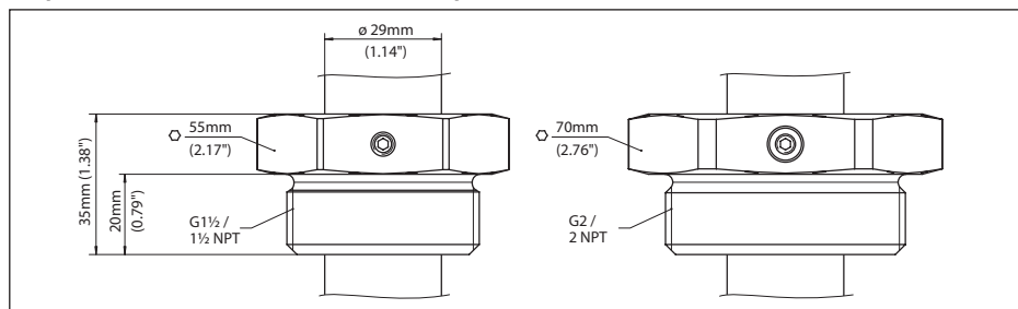
Figura 2: Dispositivo di blocco a vite ARV-VB63.1 in assenza di pressione per VEGAVIB 63
