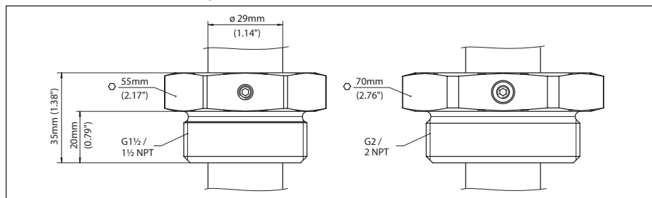
Fig. 2: Raccord d'arrêt ARV-VB63.1 sans pression pour VEGAVIB 63
