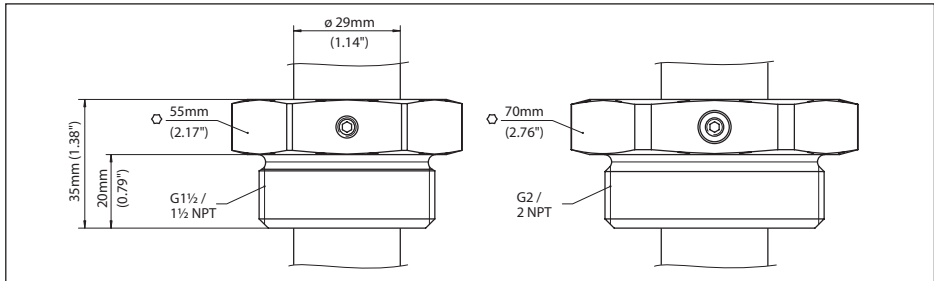
Res. 2: Basınçsız VEGAVIB 63 için durdurma dişlisi ARV-VB63.1
