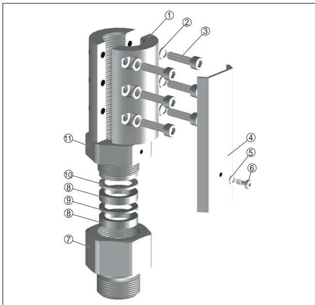
Figura 1: Dispositivo di blocco a vite ARV-SG63.3 - fino a 64 bar (928 psig)
