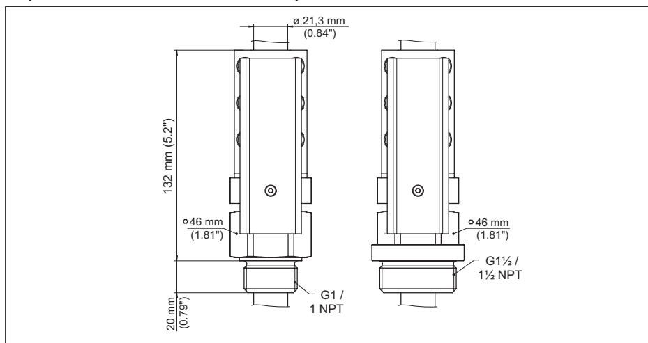
Figura 2: Dispositivo di blocco a vite ARV-SG63.3 fino a 64 bar (928 psig) per VEGASWING 63
