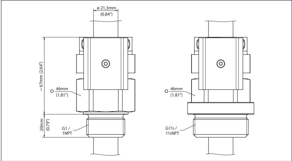
Fig. 2: Racor de retención ARV-SG63.2 hasta 16 bar (232 psig) para VEGASWING 63
