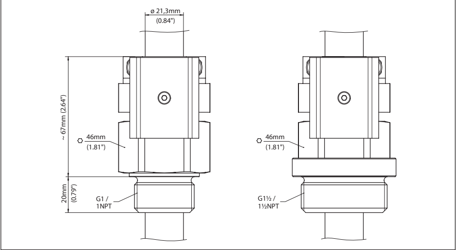
Res. 2: VEGASWING 63 için durdurma dişlisi ARV-SG63.2, 16 bar (232 psig)'a kadar
